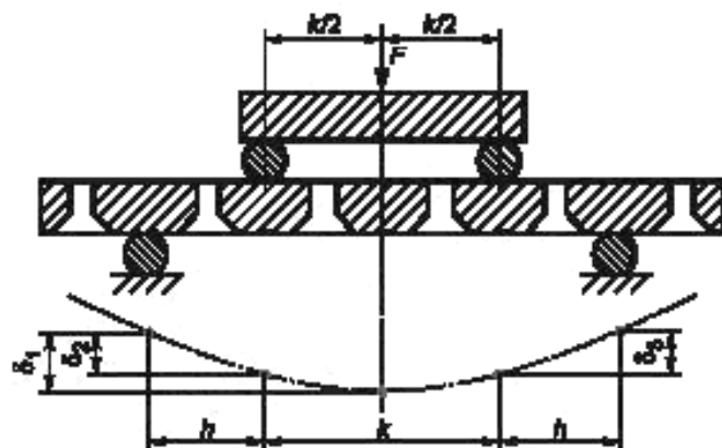
Рисунок 1 — Схема приспособления с четырьмя опорами для испытания на прочность при изгибе (внешний вид образца при изгибе)
