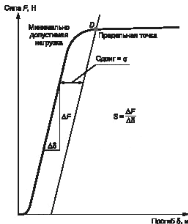
Рисунок 2 — График зависимости прогиба от нагрузки
