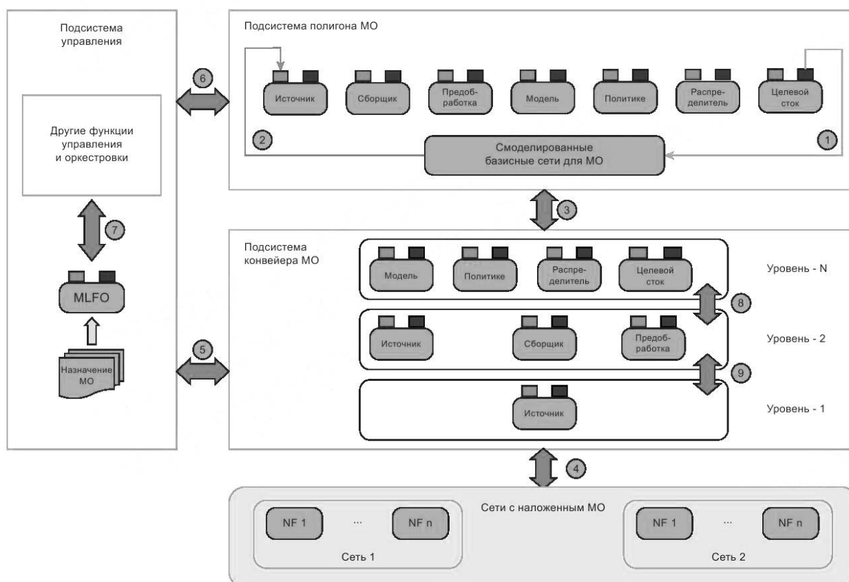
Рисунок 4 — Высокоуровневая архитектура
