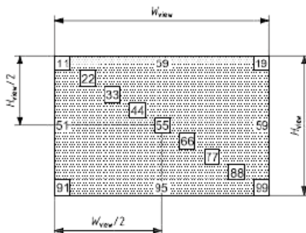
Рисунок 34 – Одиннадцать стандартных точек измерения
