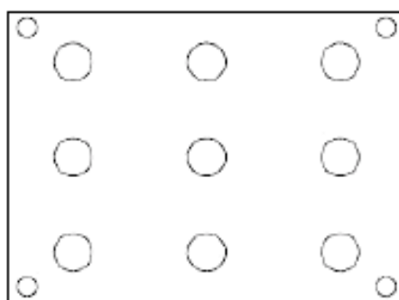
Рисунок 35 – Тринадцать стандартных точек измерения
