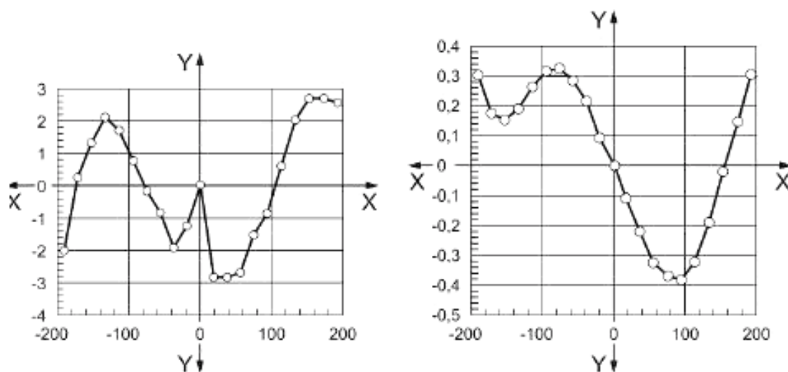
а) Линейность по горизонтали б) Погрешность позиции пикселя по горизонтали
