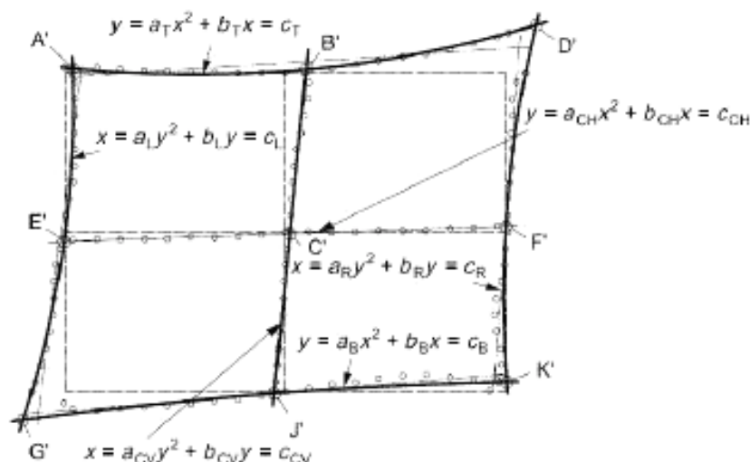
Рисунок 69 – Анализ подушкообразного искажения
