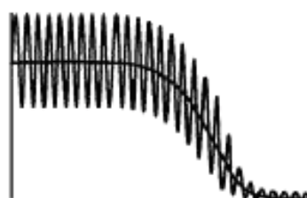
Рисунок 51– Кривая переходной характеристики с периодической пульсацией
