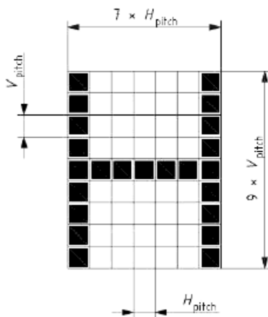
Рисунок 13 – Полноэкранный знак Н
