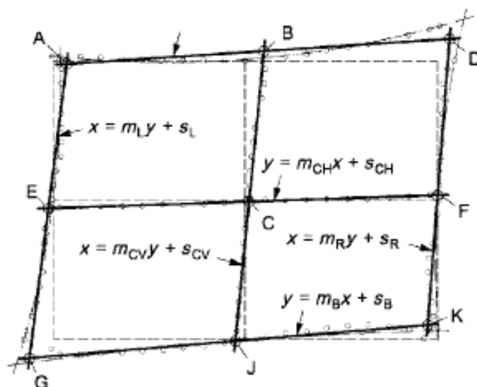
Рисунок 68 – Анализ искажений линии и испытательные позиции
