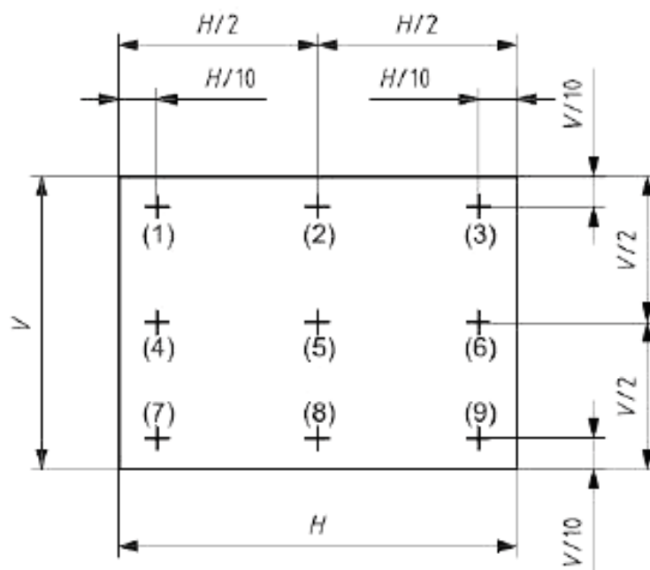
Рисунок 37 – Альтернативное расположение девяти точек измерения (VESA)
