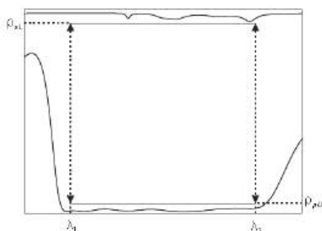
Рисунок 9 – Поляризующая функция
