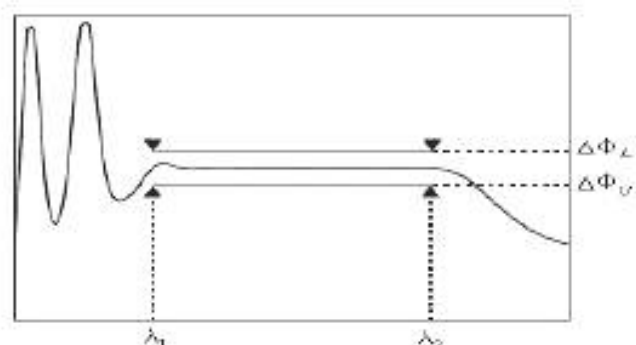
Рисунок 10 – Функция, изменяющая фазу \Delta\Phi_U, \Delta\Phi_L
