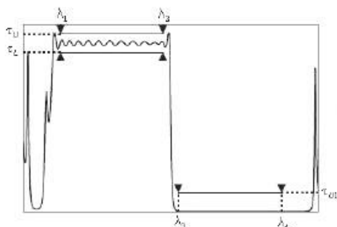
Рисунок 8 – Избирательная (комбинирующая) функция в коротковолновой области спектра
