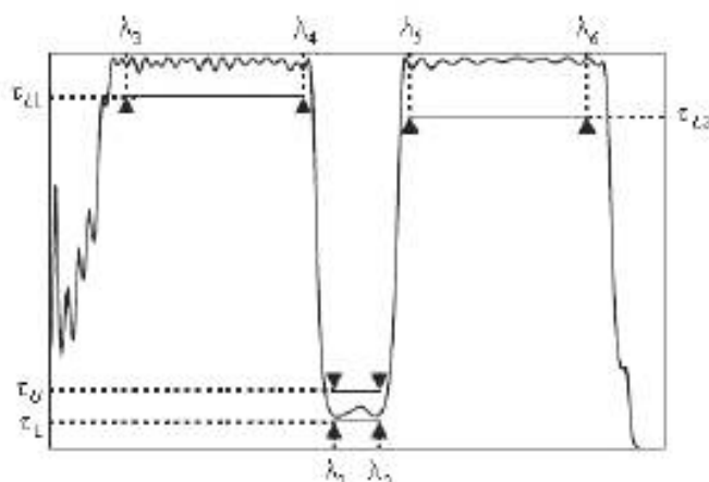
Рисунок 6 – Заграждающая функция
