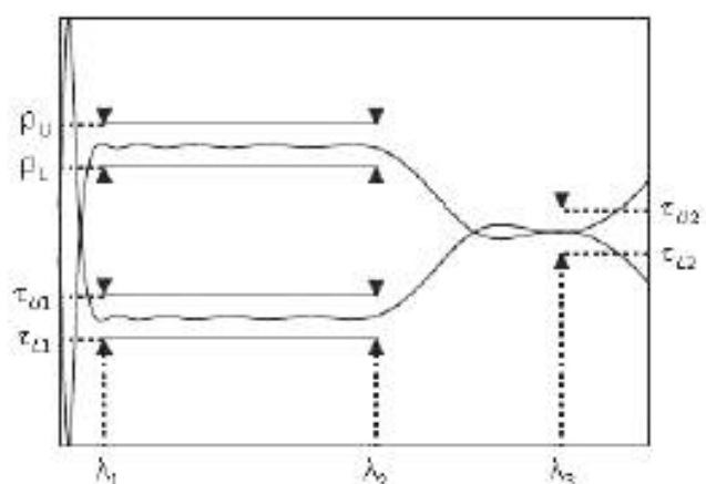
Рисунок 3 – Светоделительная функция
