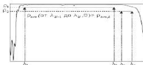
Рисунок 1 – Отражающая функция
