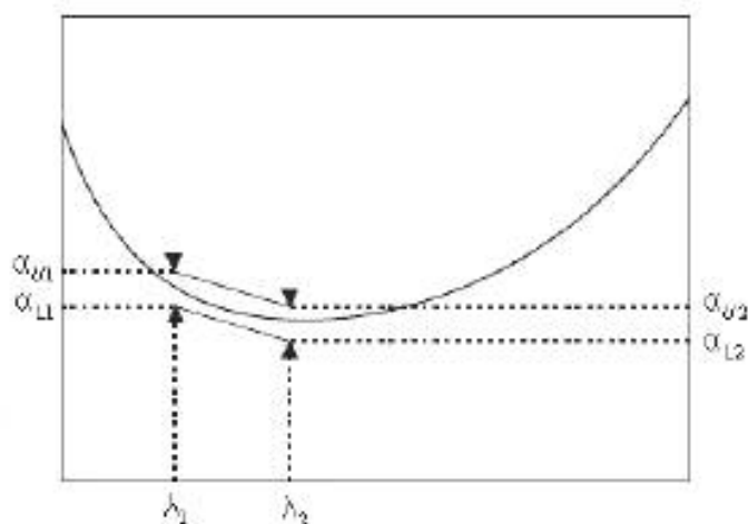
Рисунок 11 – Поглощающая функция
