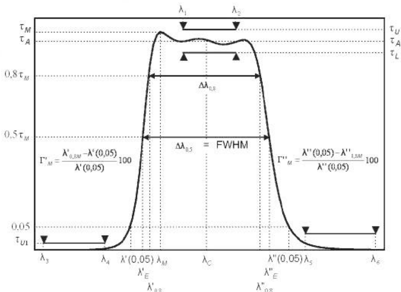
А.1 – Функция фильтрации (используется полоса пропускания \tau_M )
