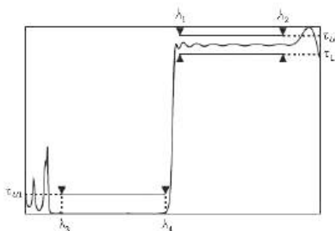
Рисунок 7 – Избирательная (комбинирующая) функция в длинноволновой области спектра
