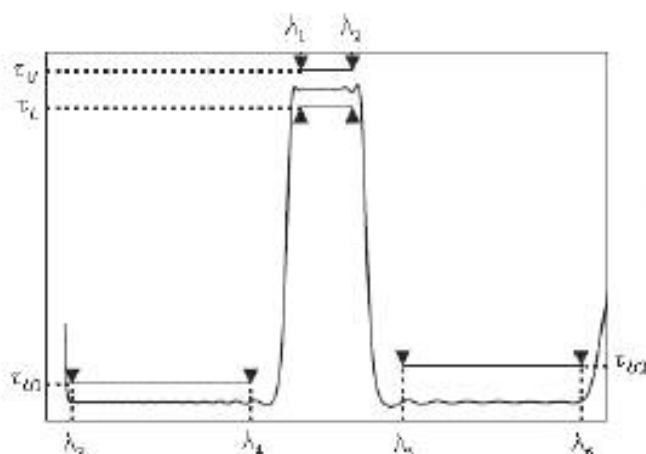
Рисунок 5 – Пропускающая функция
