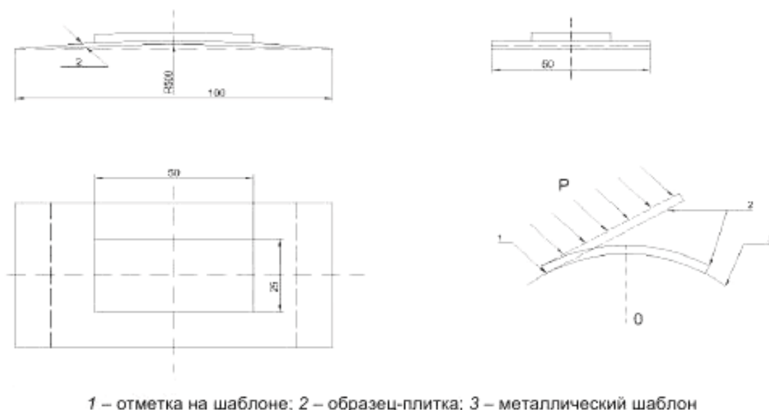
Рисунок 1 – Схема испытания на трещиностойкость
