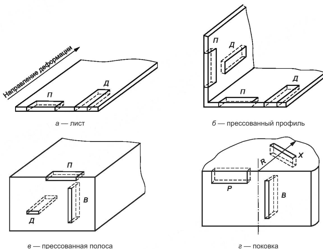
Рисунок А.1 — Схемы вырезки образцов
