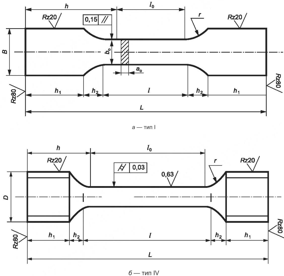
Рисунок Б.1 — Форма и размеры образцов для испытаний при постоянной осевой нагрузке и при деформации с малой постоянной скоростью
