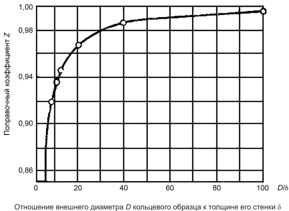
Рисунок Г.1 — График зависимости поправочного коэффициента от отношения внешнего диаметра кольцевого образца к толщине его стенки
