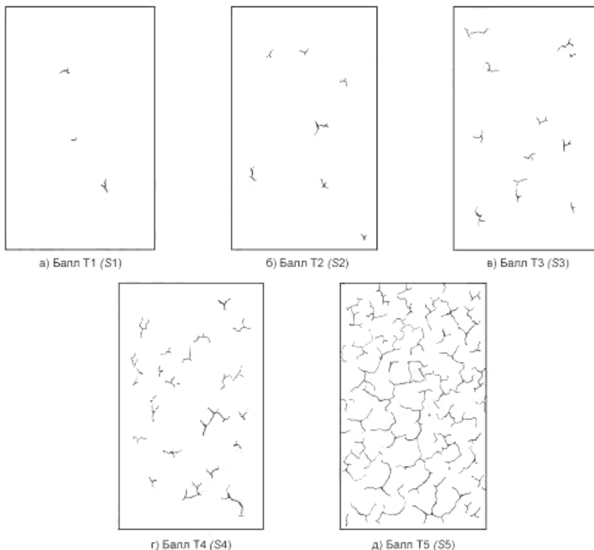
Рисунок 1 — Растрескивание без предпочтительного направления (площадь осматриваемой поверхности от 1 дм 2 до 2 дм 2 )
