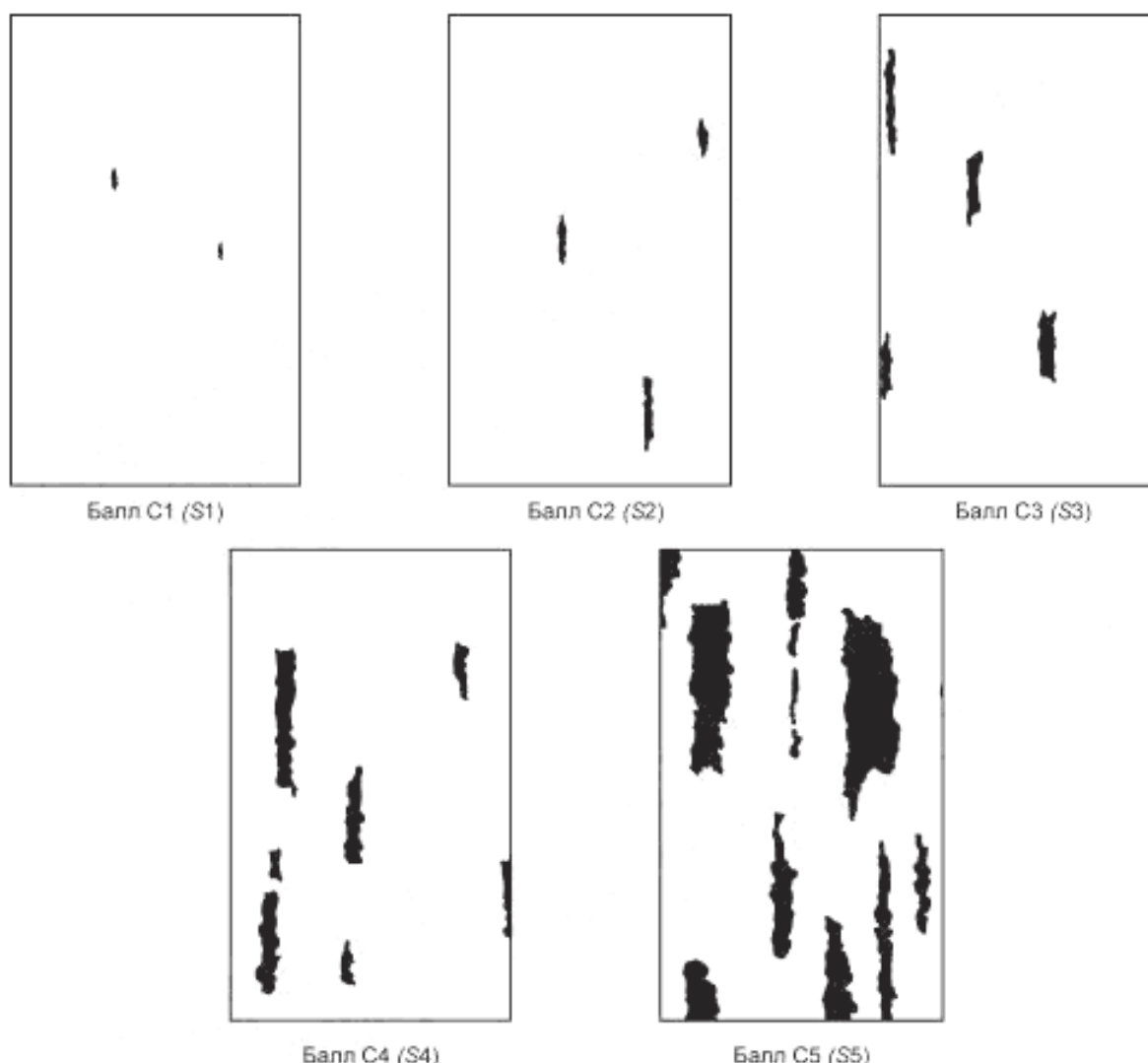
Рисунок 4 — Отслаивание в одном предпочтительном направлении (площадь осматриваемой поверхности от 1 дм 2 до 2 дм 2 )
