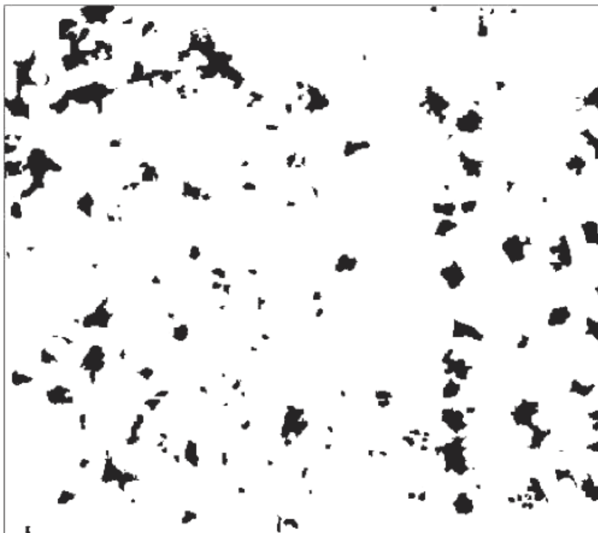
Рисунок Ж.4 — Коррозия металла, балл К4 (или R i 4)
