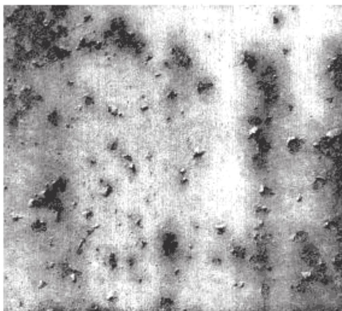
Рисунок 12 — Коррозия металла балл К4 (или R4)
