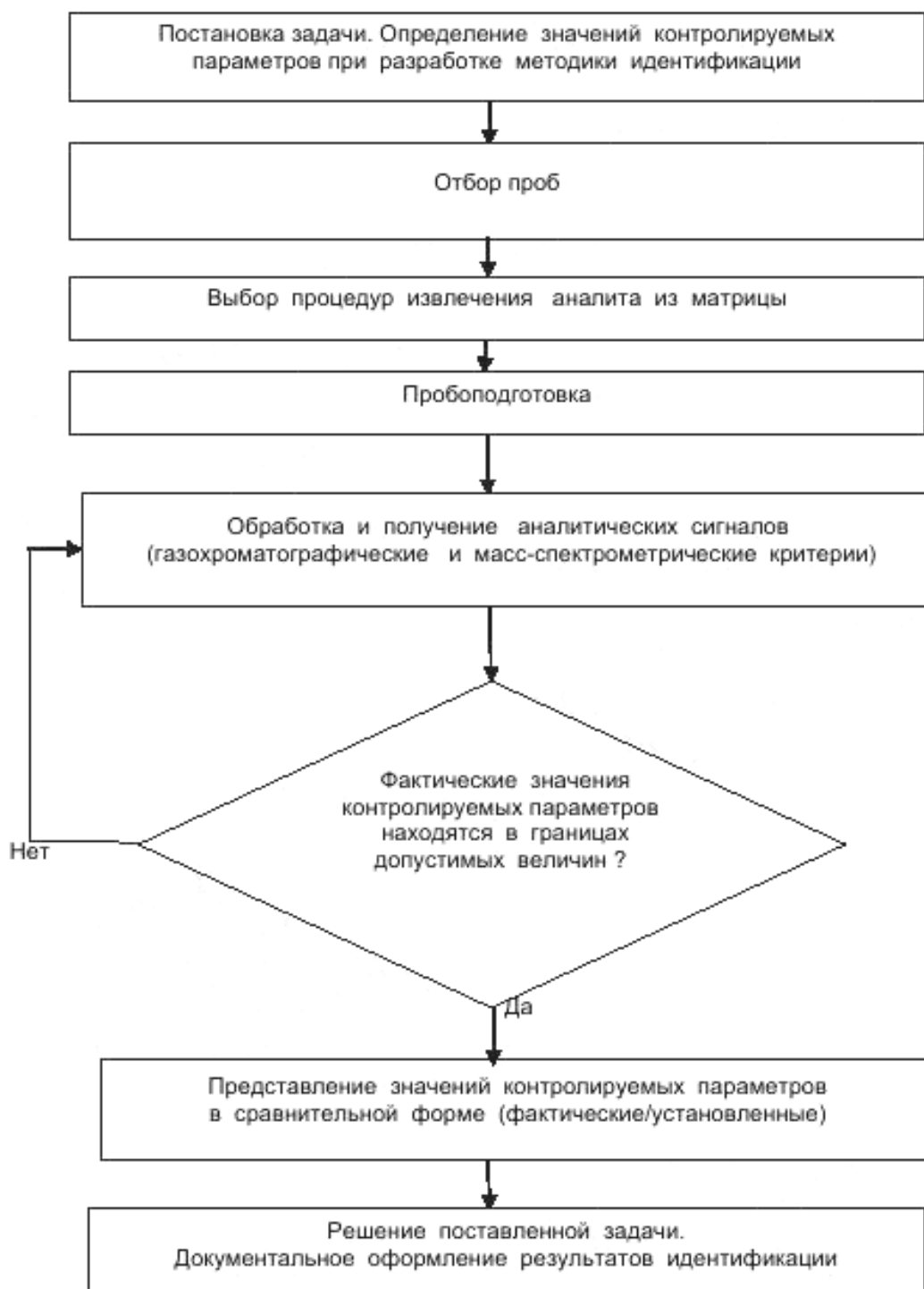
Рисунок 1 – Блок-схема идентификации
