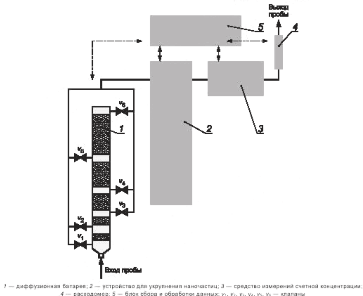
Рисунок 1 — Типичная блок-схема диффузионного аэрозольного анализатора
