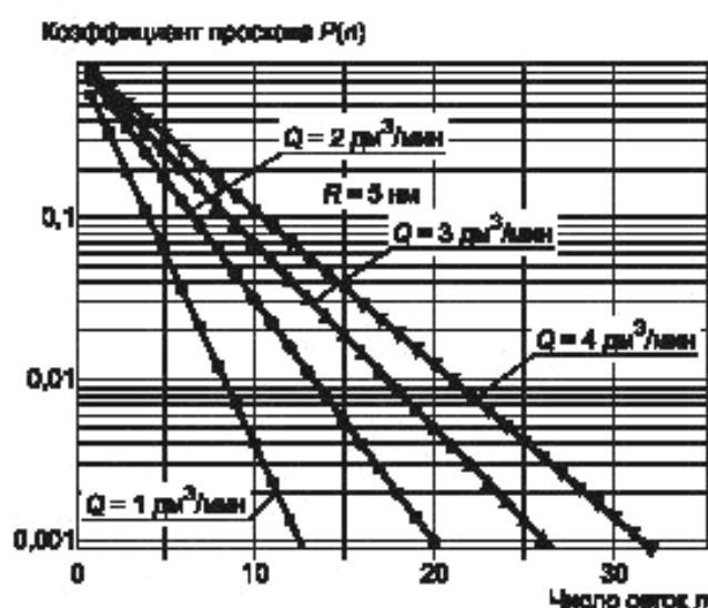
Рисунок В.1 — Зависимость коэффициента проскока аэрозольных частиц размером 10 нм от числа сеток в диффузионной батарее при объемных скоростях 1, 2, 3 и 4 \text{дм}^3/\text{мин}
