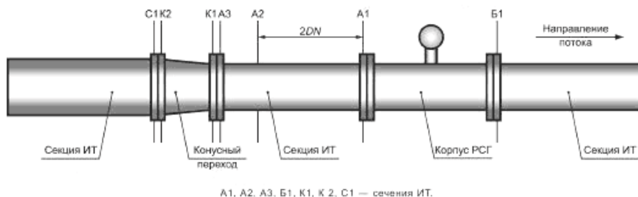
Рисунок 6 — Сечения, в которых измеряют внутренний диаметр ИТ в случае применения конусных переходов
