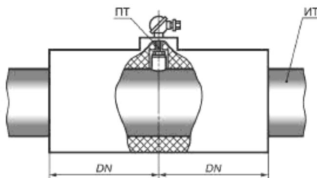
Рисунок 1 — Примеры теплоизоляции корпуса участков ИТ и ПТ
