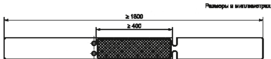
Рисунок 4 — Удлиненная балясина люцманского штурмтрапа
