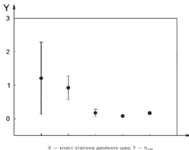
Рисунок А.13 — Соотношение между классом эталона двойного шва и разбросом высоты
