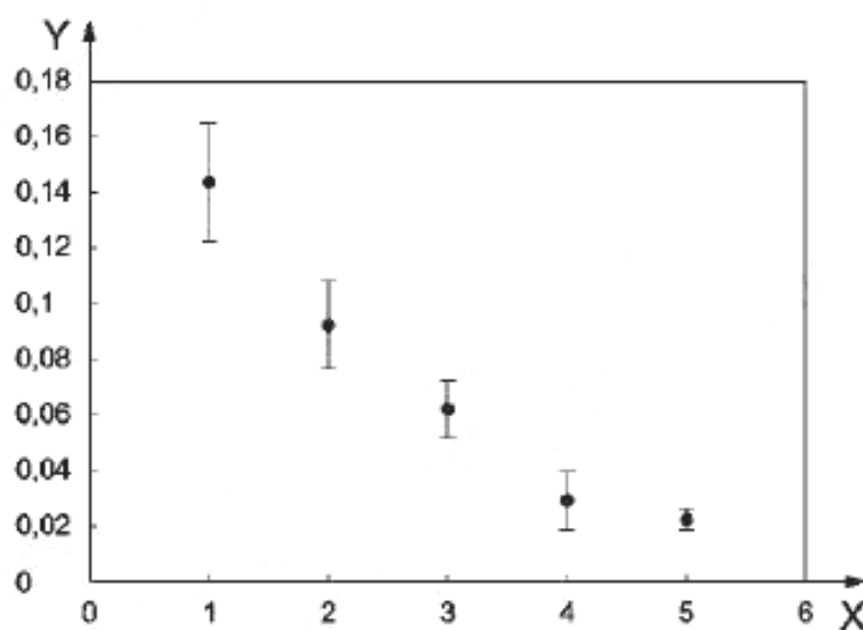
Рисунок А.7 — Соотношение между классом эталона одинарного шва и средним значением частоты высоты
