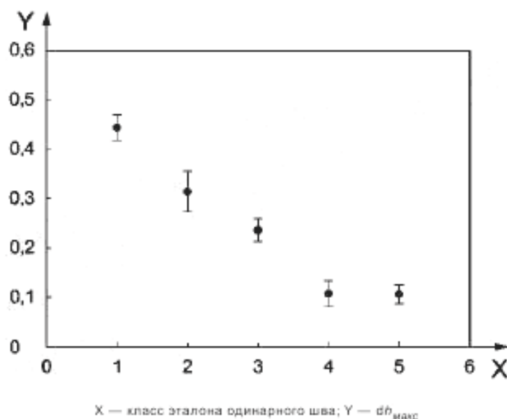
Рисунок А.8 — Соотношение между классом эталона одинарного шва и максимальным значением частоты высоты
