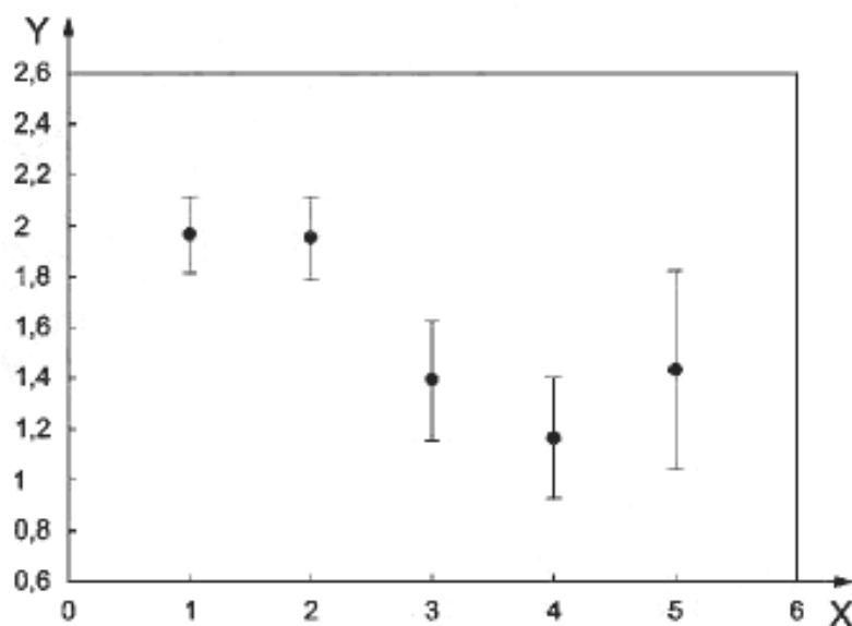
Рисунок A.4 — Соотношение между классом эталона одинарного шва и средним значением высоты
