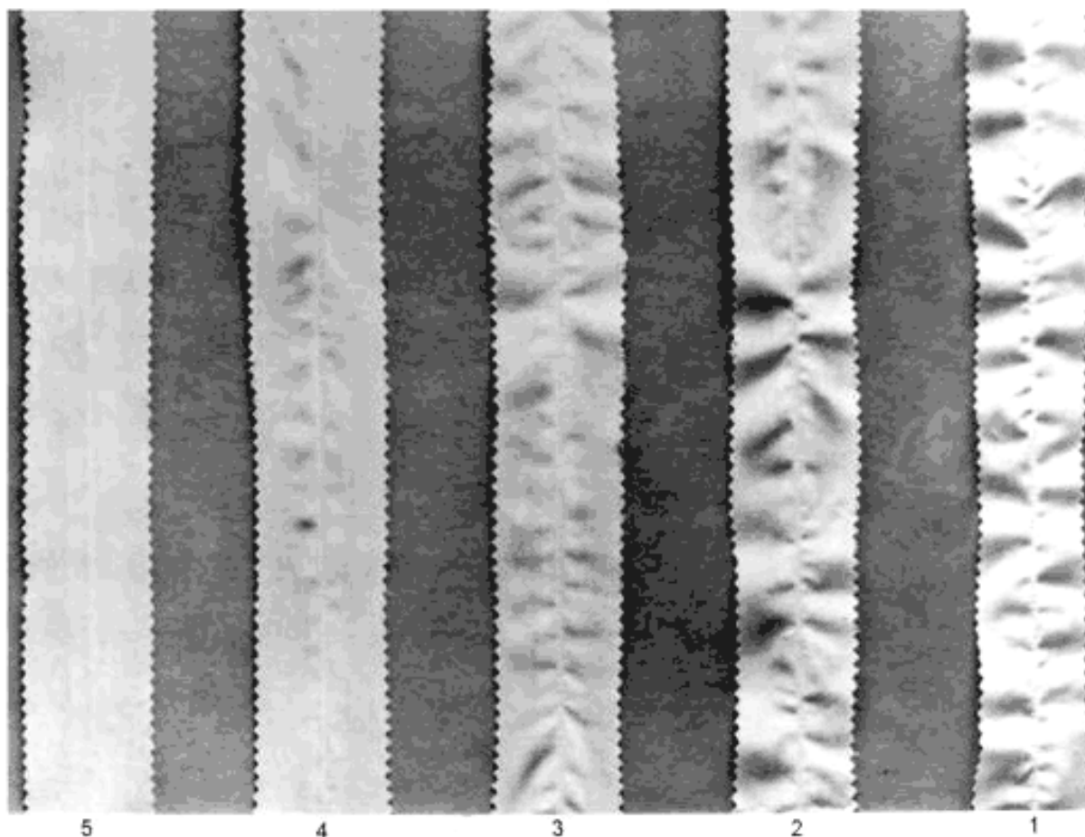
Рисунок 2 — Фотография сравнительной шкалы для одинарных швов
