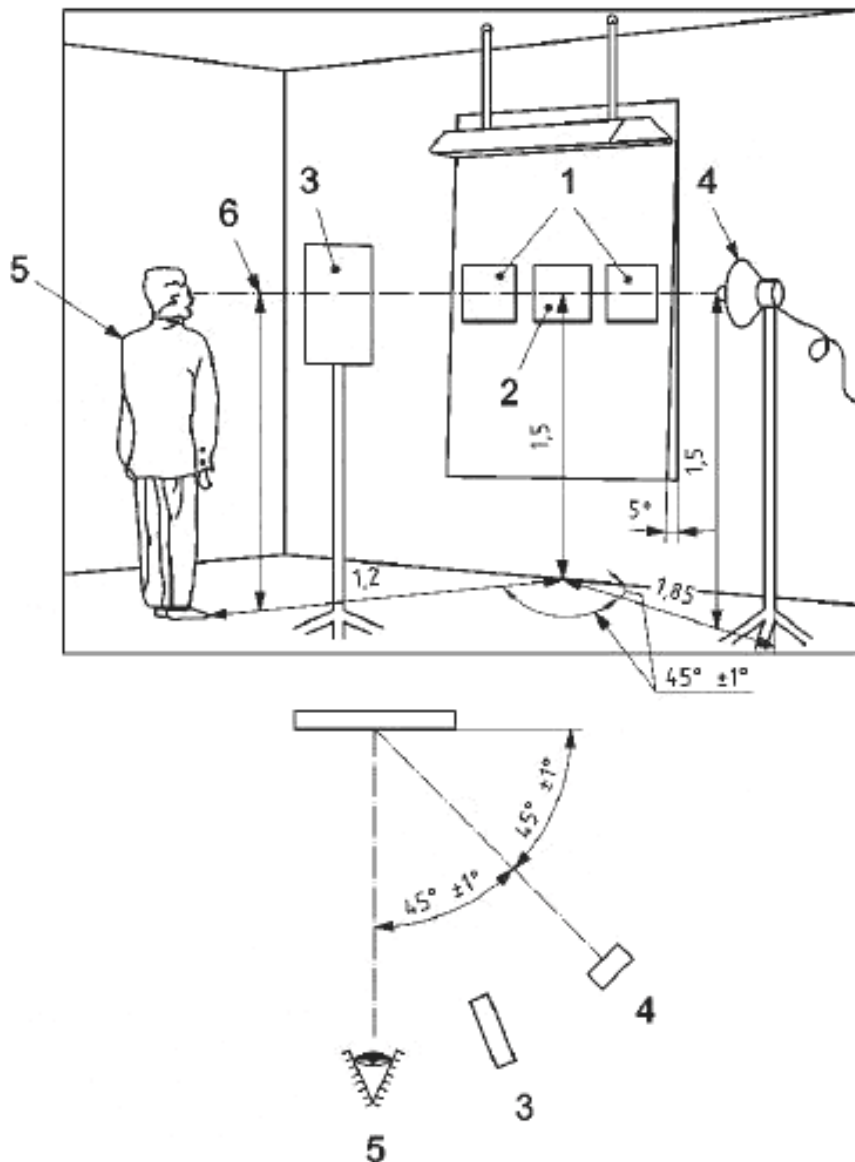
1 — эталон; 2 — образец для испытаний; 3 — экранирующая блenda; 4 — 500-ваттная лампа-рефлектор; 5 — эксперт; 6 — произвольно выбранный уровень глаз
