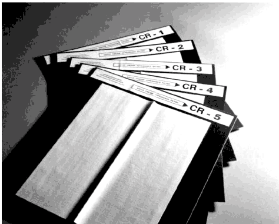
Рисунок 3 — Пластмассовые эталоны складок
