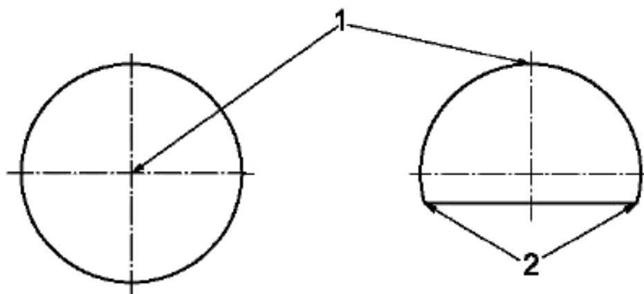
Рисунок А.1 — Расположение точек на сферической головке
