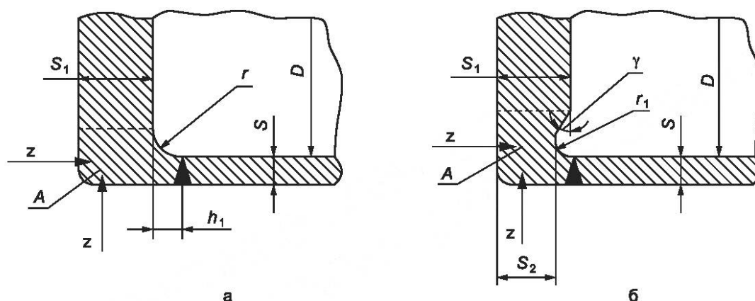
D — внутренний диаметр обечайки; S — толщина обечайки; S_1 — толщина фланца; S_2 — наименьшая толщина фланца в месте кольцевой выточки; h_1 — длина отбортовки фланца; r — радиус закругления фланца; r_1 — радиус кольцевой выточки; \gamma — угол проточки фланца
