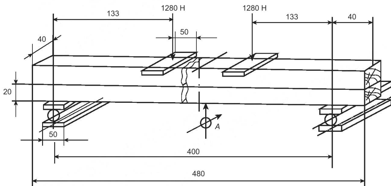
Рисунок 4 — Схема испытания
