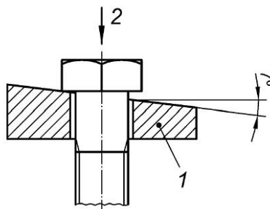
1 — клиновидная шайба; 2 — сила сжатия
