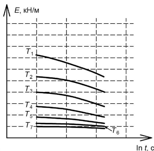
Рисунок Г.2 — Податливость в полулогарифмической системе координат
