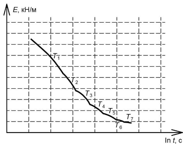
Рисунок Г.3 — Смещенные кривые податливости
