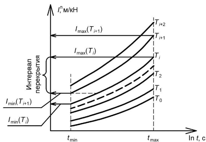
Рисунок В.2 — Графическое изображение экспериментальных данных в координатах I^n — \ln t и схема определения коэффициента перекрытия — k_n кривых вязкоупругой податливости
