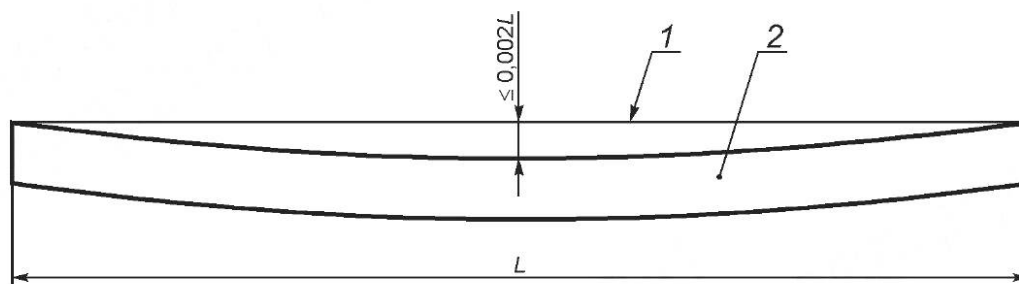
Рисунок 1 — Измерение общей прямолинейности
