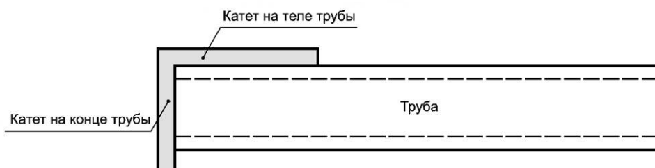
Рисунок 3 — Схема измерения прямоугольником
