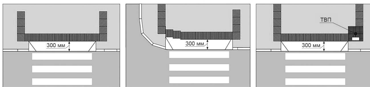
Рисунок Б.14 — Пример обустройства пешеходного перехода сигнальными пластинами на улицах с четырьмя полосами движения
