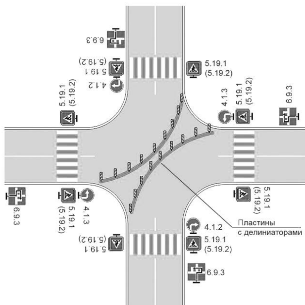
б) Установка делиниаторов и дорожных пластин
