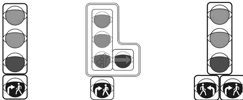
Рисунок Б.4 — Информационная световая секция, примеры размещения со светофором
