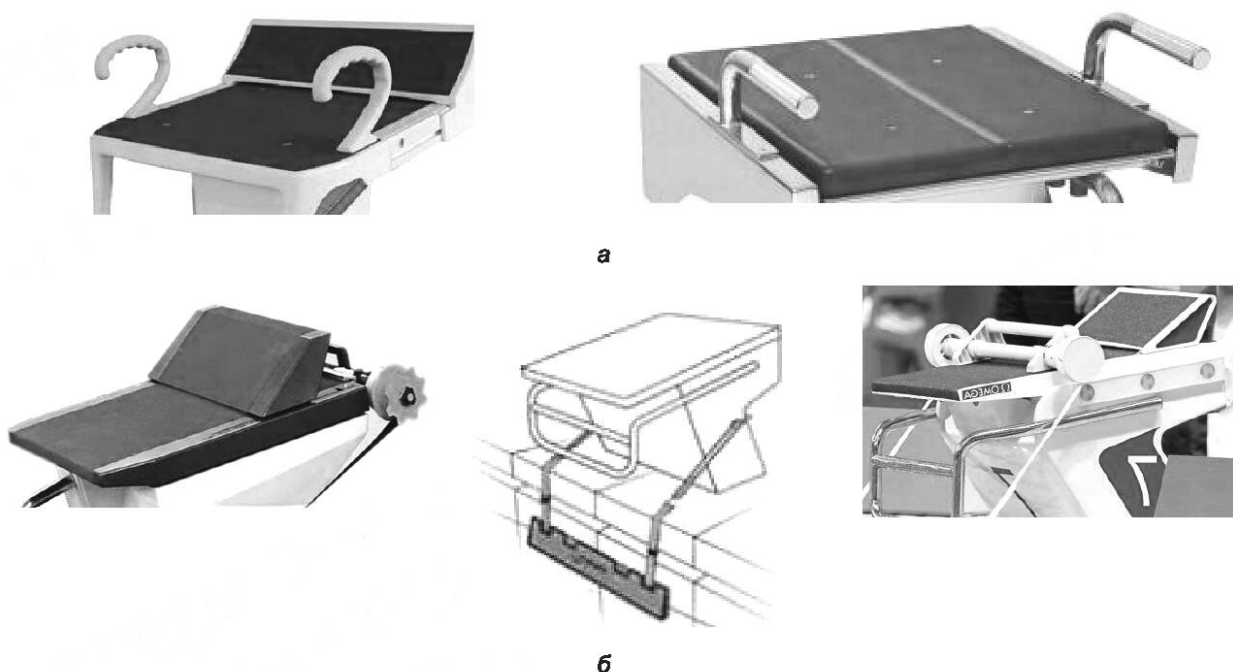
а — хватыв для рук и упор на стартовой поверхности соревновательных тумб; б — крепление планки для старта в плавании на спине (нижний регулируемый упор)
