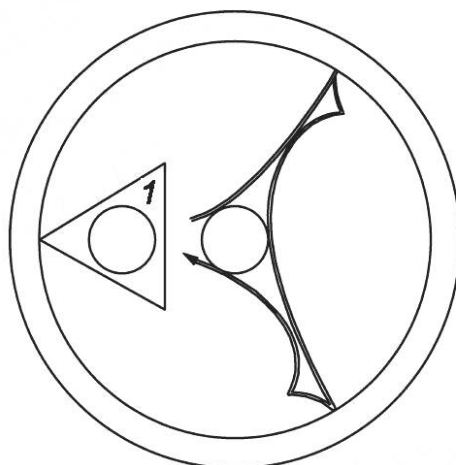
1 — роликовый узел
