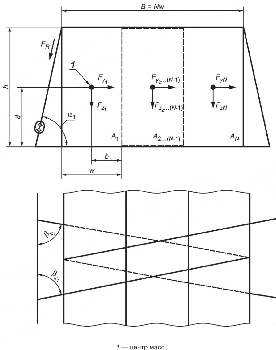
Рисунок 13 — Расчетная схема при креплении петель для предотвращения опрокидывания одного или нескольких рядов груза
