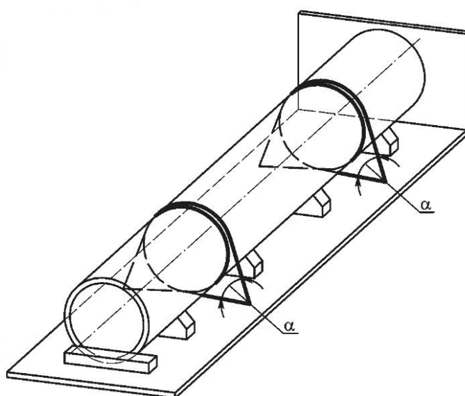
Рисунок 11 — Крепление петель
