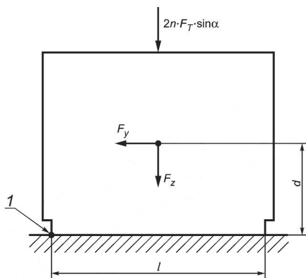
1 — ребро опрокидывания
