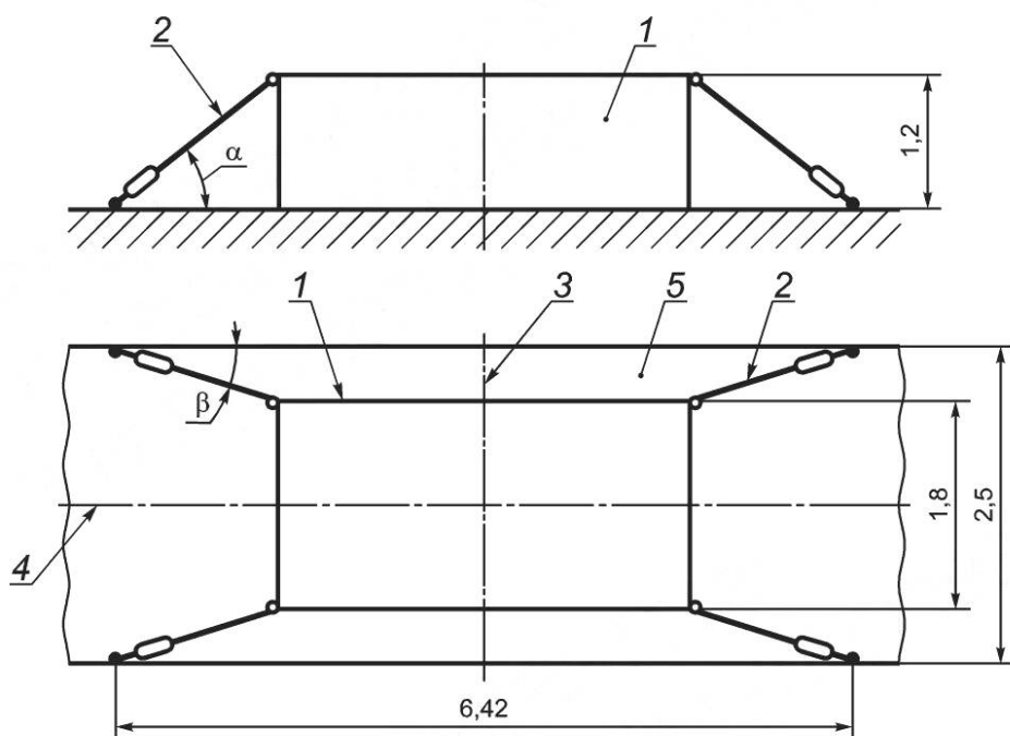
Рисунок Г.1 — Расчетная схема для прижимного натяжения гибкого средства крепления
