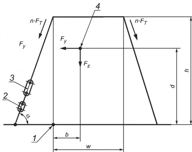
Рисунок 4 — Расчетная схема при прижимном натяжении гибких средств крепления для предотвращения опрокидывания груза в поперечном направлении
