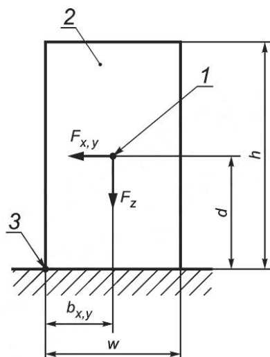
1 — центр масс; 2 — груз; 3 — ребро опрокидывания
