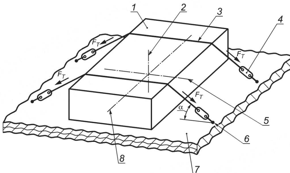
1 — груз; 2 — вертикальная ось; 3 — гибкое средство крепления; 4 — натяжное устройство; 5 — поперечная ось; 6 — точка крепления; 7 — горизонтальная плоскость загрузки (поверхность, с которой соприкасается груз); 8 — продольная ось
