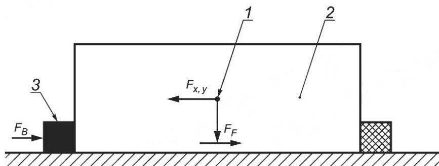
1 — центр масс; 2 — груз; 3 — ребро опрокидывания
