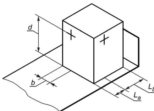
Рисунок 17 — Грузовая единица или секция груза с центром масс, удаленным от геометрического центра этой грузовой единицы или секции груза
