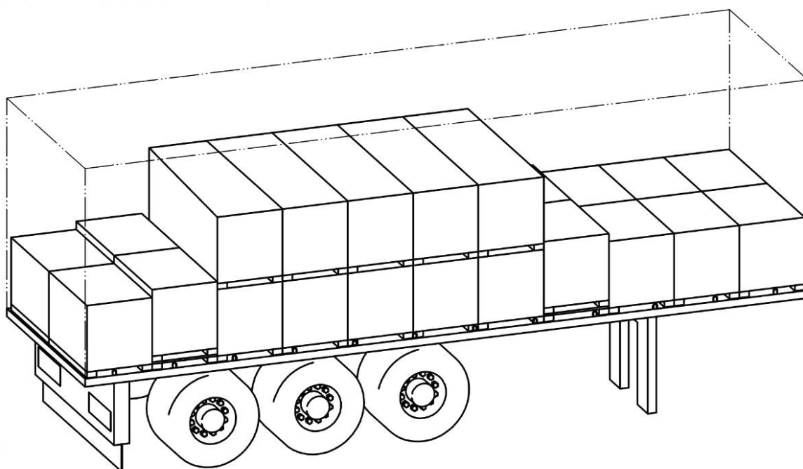
Рисунок Г.3 — Загрузка полуприцепа
