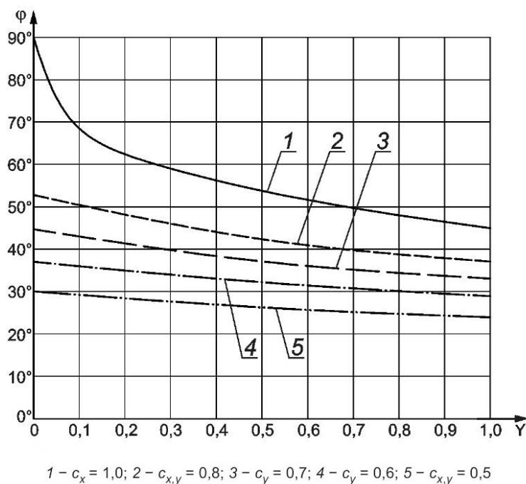
Рисунок 18 — Диаграмма для определения значения угла наклона грузовой платформы \varphi
