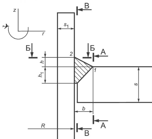
Рисунок А.3 — Схематизация фрагмента МК РБМК-1000 в районе штуцерного сварного соединения (вварки трубы тракта в плиту)
