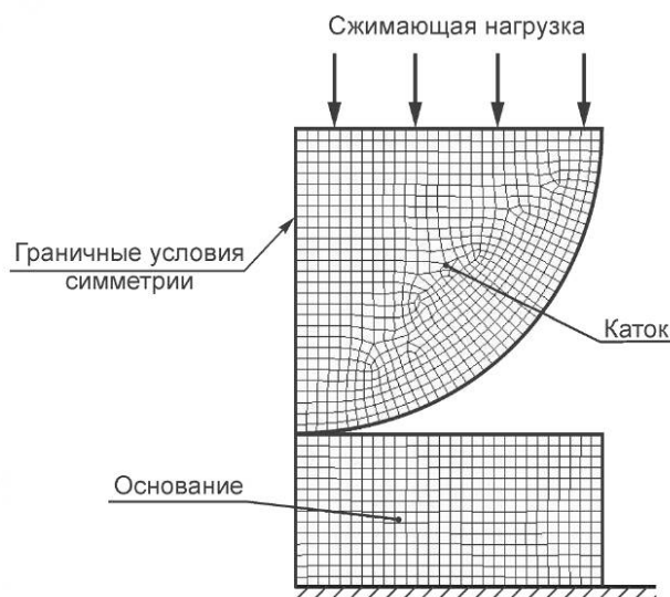
Рисунок Б.1 — Пример расчетной схемы катковой опоры
