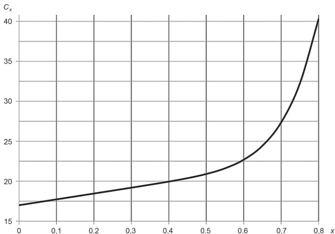
Рисунок 9.1 — График для определения C_x
