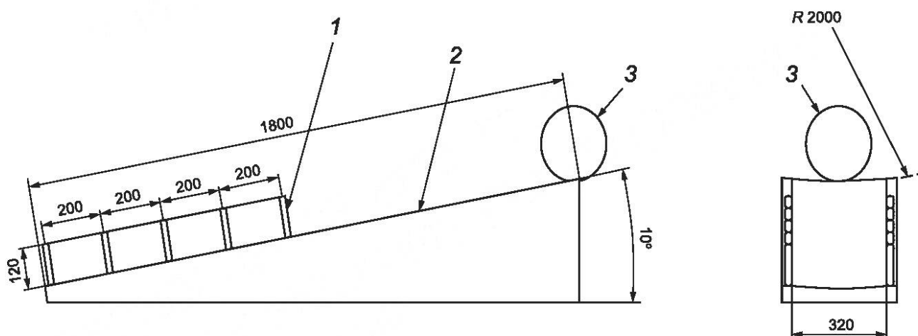
1 — штанга-ограничитель; 2 — наклонная поверхность; 3 — мяч
