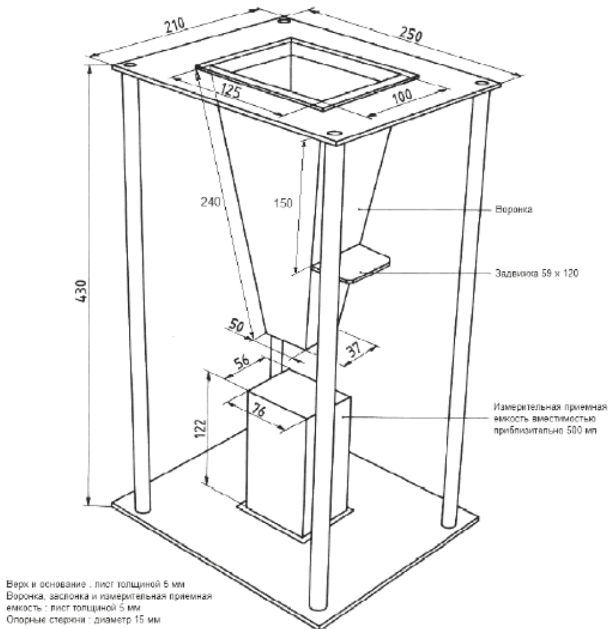
Рисунок 1 – Устройство для определения объемной плотности
