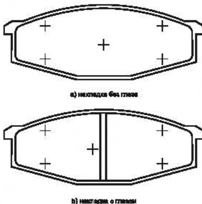
Рисунок 3 — Указания по измерению толщины образца
