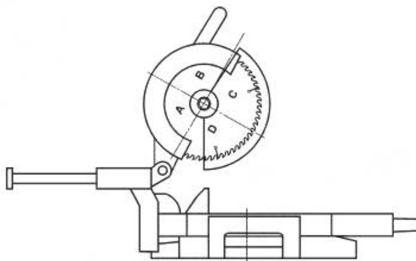
б) Торцовочная пила в крайнем верхнем положении
