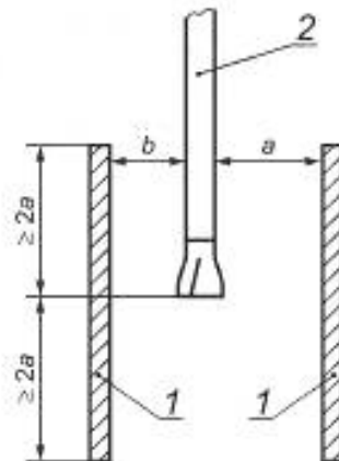
a , b — расстояния между плоскостью пильного диска и внутренней поверхностью бокового барьера; 1 — боковая стенка; 2 — пильный диск.
