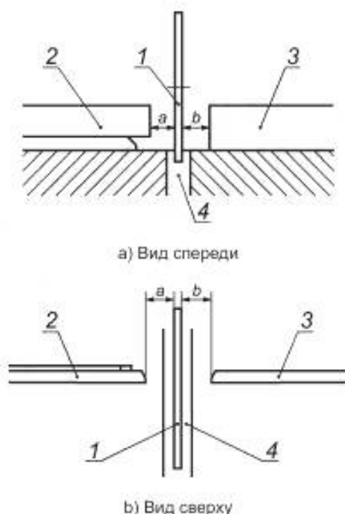
Рисунок 110 — Расстояние между упором и пильным диском
