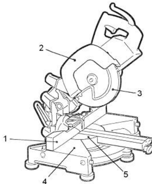
1 — упор; 2 — верхний защитный кожух; 3 — нижний защитный кожух; 4 — основание стола; 5 — поворотный стол
