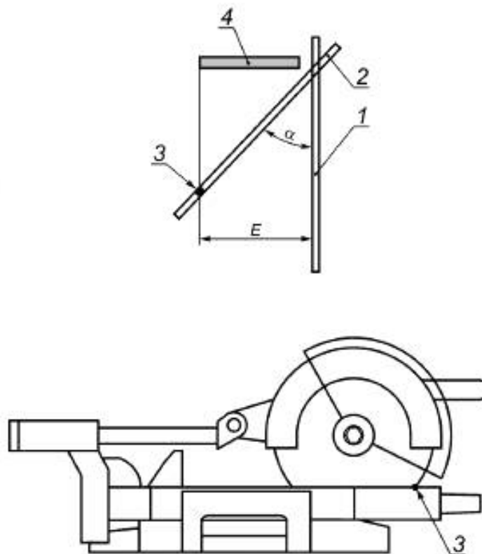
\alpha — максимальный угол скоса (показано резание слева); E — минимальное удлинение упора (см. 21.103); 1 — стальной диск при угле наклона диска 0^\circ и угле скоса 0^\circ ; 2 — стальной диск при угле наклона диска 0^\circ и максимальном угле скоса; 3 — точка пересечения стального диска с рабочей поверхностью стола при угле наклона диска 0^\circ и максимальном угле скоса; 4 — упор
