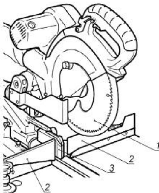
1 — пильный диск; 2 — упоры; 3 — центральная поддержка объекта обработки
