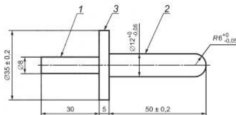
1 — участок рукоятки; 2 — испытательный участок; 3 — фланец щупа
