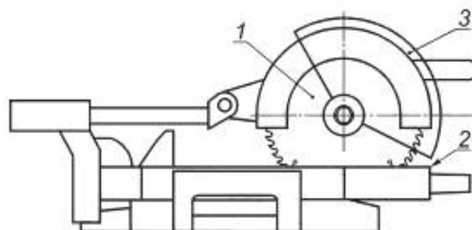
1 — пильный диск; 2 — конец стола; 3 — нижний защитный кожух
