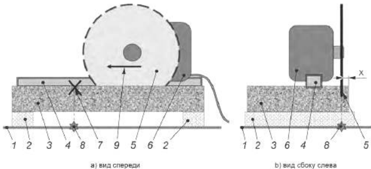
1 — основание (отражающая плоскость); 2 — упор; 3 — бетонный объект обработки; 4 — система направляющих; 5 — алмазный круг; 6 — пильная головка; 7 — средняя точка реза, выполненного во время измерения; 8 — центр полусферы радиусом R ; 9 — направление резания
