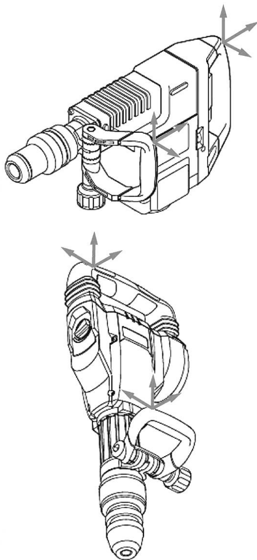
Рисунок I.105 — Место установки измерительного преобразователя для молотков
