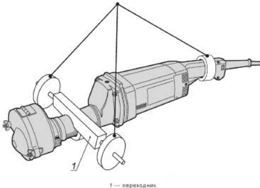
Рисунок 112 — Испытание кожуха на прочность: прямая шлифовальная машина с дополнительными массами
