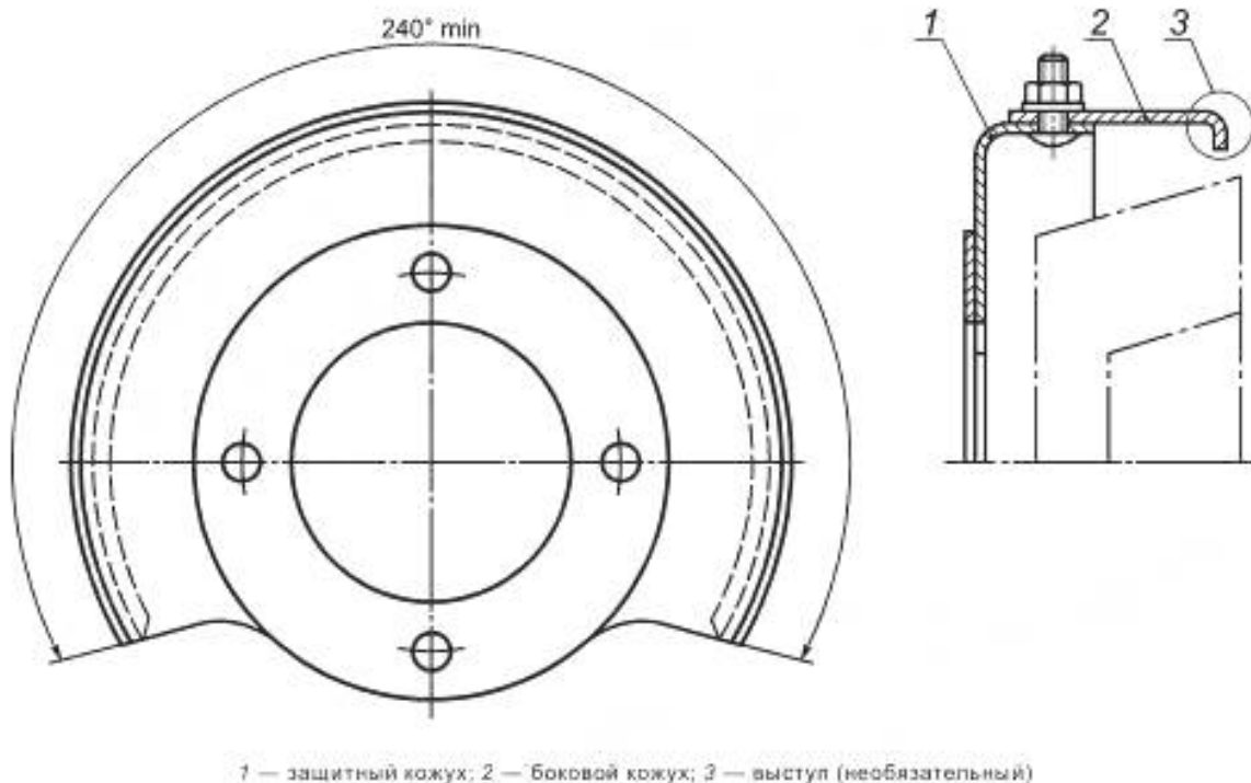
Рисунок АА.4 — Регулируемый защитный кожух типа D
