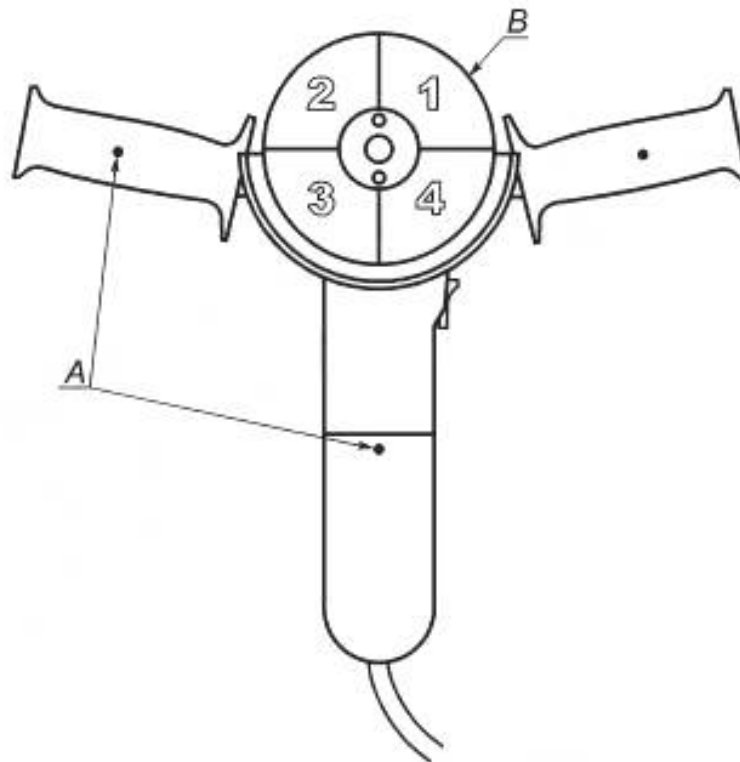
Рисунок 108 — Испытание кожуха на прочность: подготовка шлифовальной машины
