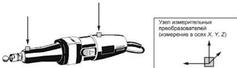
Рисунок I.101 — Расположение измерительных преобразователей для прямых шлифовальных машин
