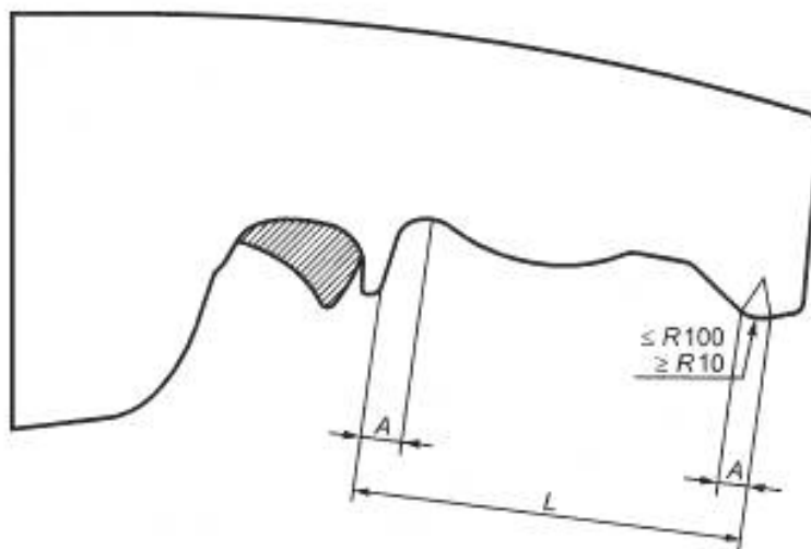
Рисунок 114 — Измерение длины поверхности захвата рукоятки
