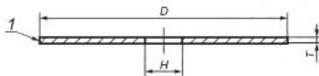
Рисунок СС.8 — Круг типа 41
