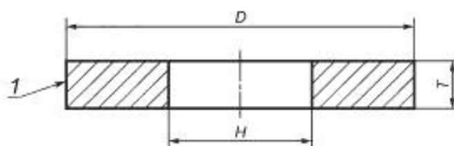
Рисунок СС.1 — Круг типа 1
