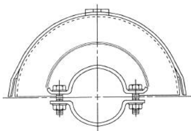
б) Защитный кожух типа G с передним ограждением
