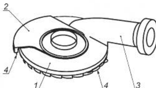
1 — защитный кожух; 2 — съёмная часть защитного кожуха для обеспечения шлифовки; 3 — средства для удаления пыли; 4 — гибкая периферийная часть защитного кожуха
