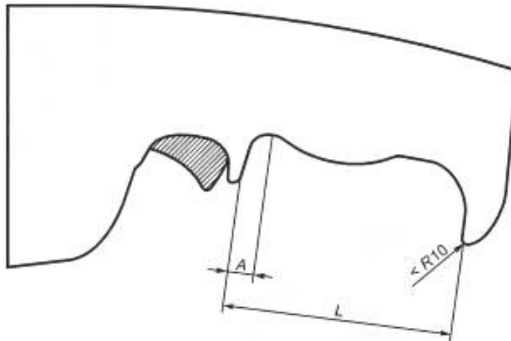
Рисунок 113 — Измерение длины поверхности захвата рукоятки
