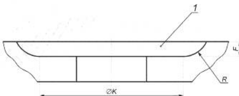
Рисунок Z101 — Углубление центра абразивных кругов
