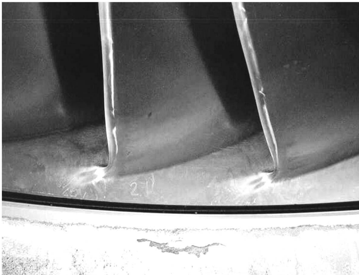
Рисунок 5 — Пример кавитации на ободу рабочего колеса из-за утолщенных лопастей
