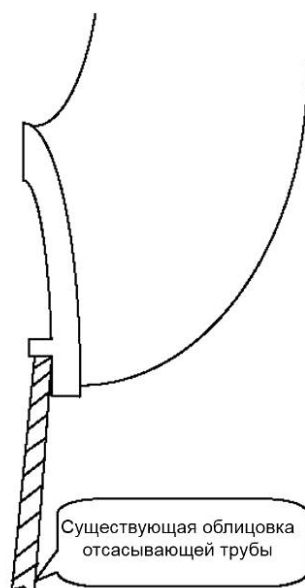
Рисунок 4 — Увеличение площади лопастей рабочего колеса при модернизации
