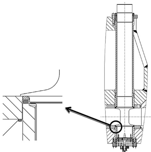
Рисунок 6 — Пример конструкции уплотнений цапф направляющей лопатки
