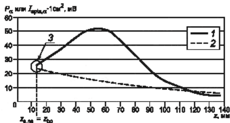
Рисунок А.5 — Фокусирующий преобразователь с апертурой, меньшей чем на рисунке А.4
