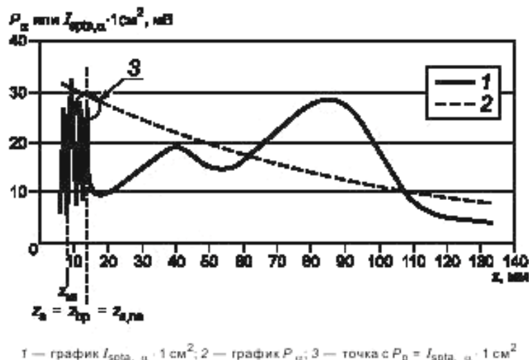
Рисунок А.3 — Фокусирующий преобразователь (число f \geq 10 ) с сильными пространственными флуктуациями вблизи излучающей поверхности
