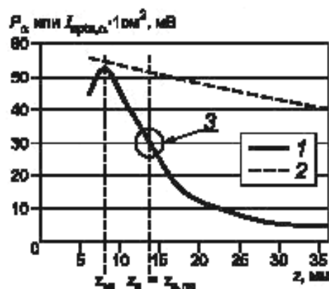
1 — график I_{spta, \alpha} \times 1 \text{ см}^2 ; 2 — график P_a ; 3 — точка с P_a = P_a(z_s, ns) z_{Ml} расположен ближе к преобразователю, чем 1,5 \cdot D_{eq}
