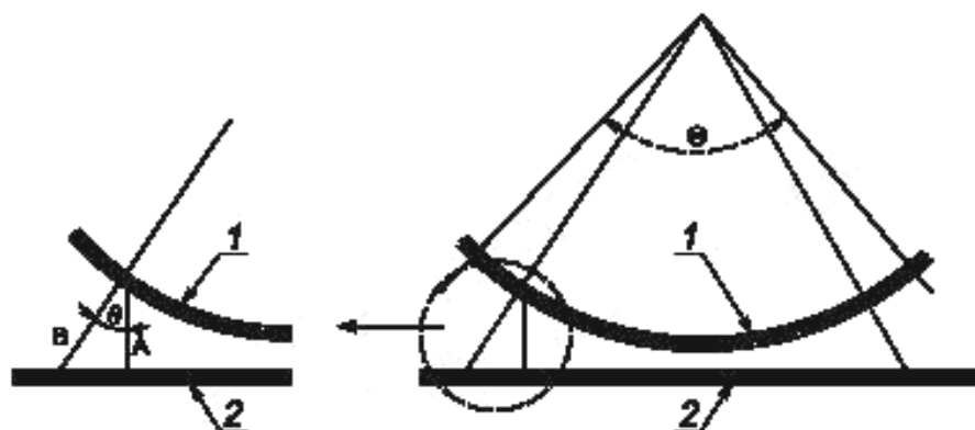
1 — решетка; 2 — поглощающая мишень; \Theta — угол сканирования; \varphi — угол падения
