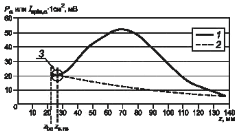
Рисунок А.4 — Фокусирующий преобразователь
