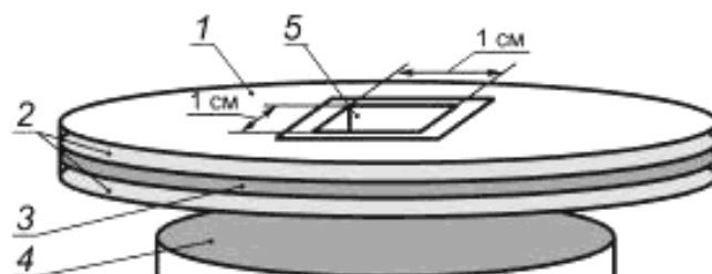
1 — отражающее покрытие; 2 — поглонитель; 3 — слой отражателя; 4 — ультразвуковой преобразователь; 5 — окно 1 × 1 см
