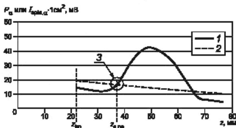
1 — график I_{spta, \alpha} \times 1 \text{ см}^2 ; 2 — график P_a ; 3 — точка, где P_a = P_a(z_s, ns) = I_{spta, \alpha} \times 1 \text{ см}^2
