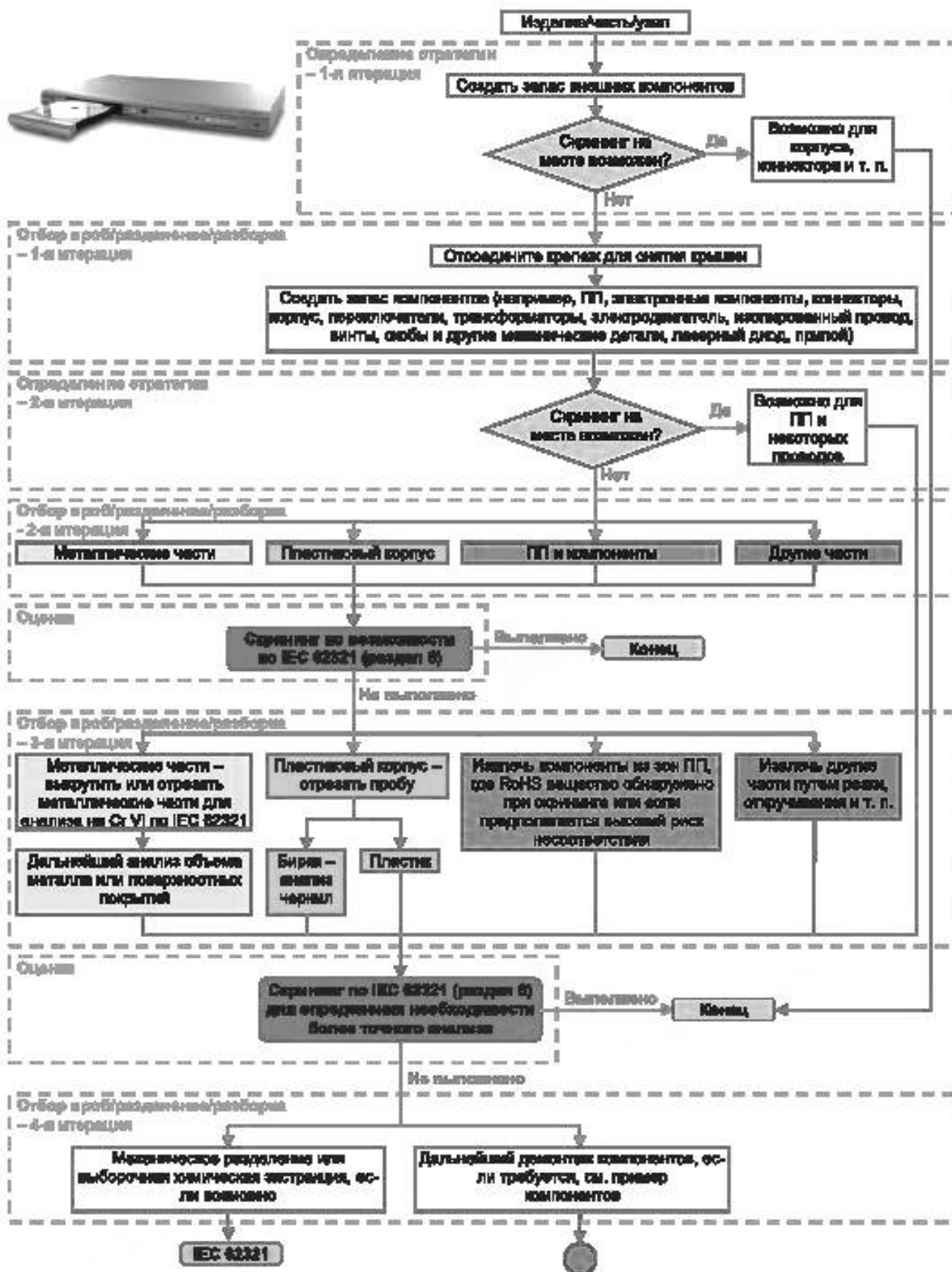
Рисунок A.2 — Отбор образцов DVD-проигрывателя
