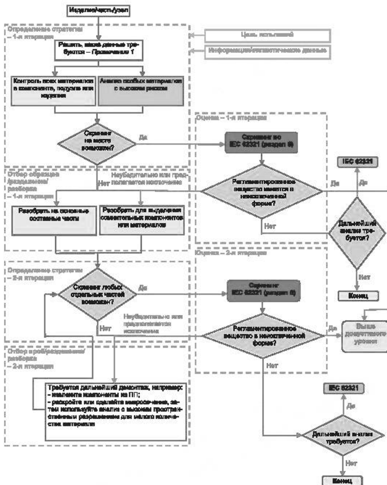
Рисунок А.1 — Методология отбора образцов и разделения
