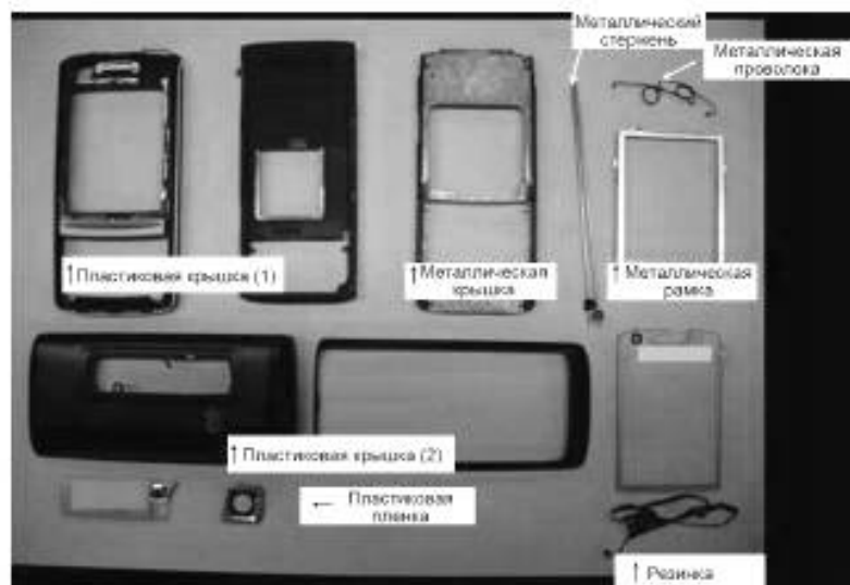
Рисунок E.6 — Полная разборка остального корпуса/рамки
