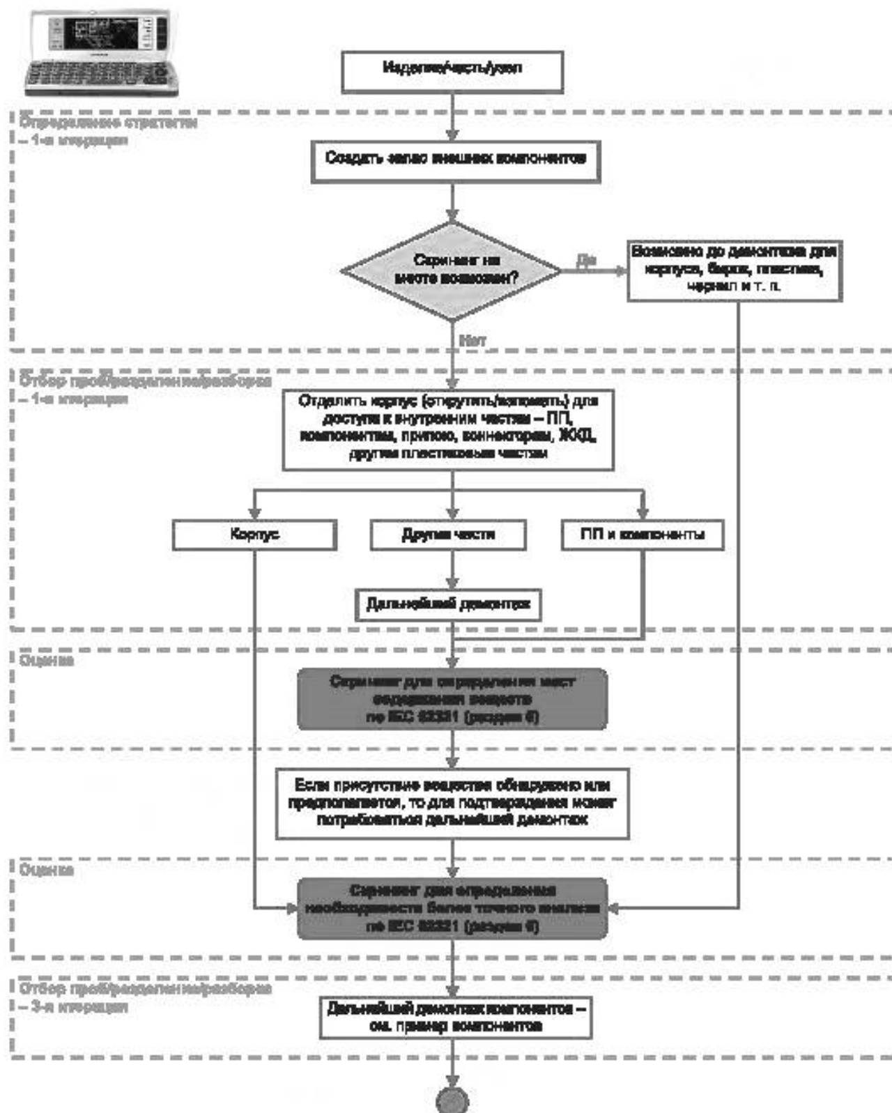
Рисунок А.5 — Отбор образцов PDA/телефона
