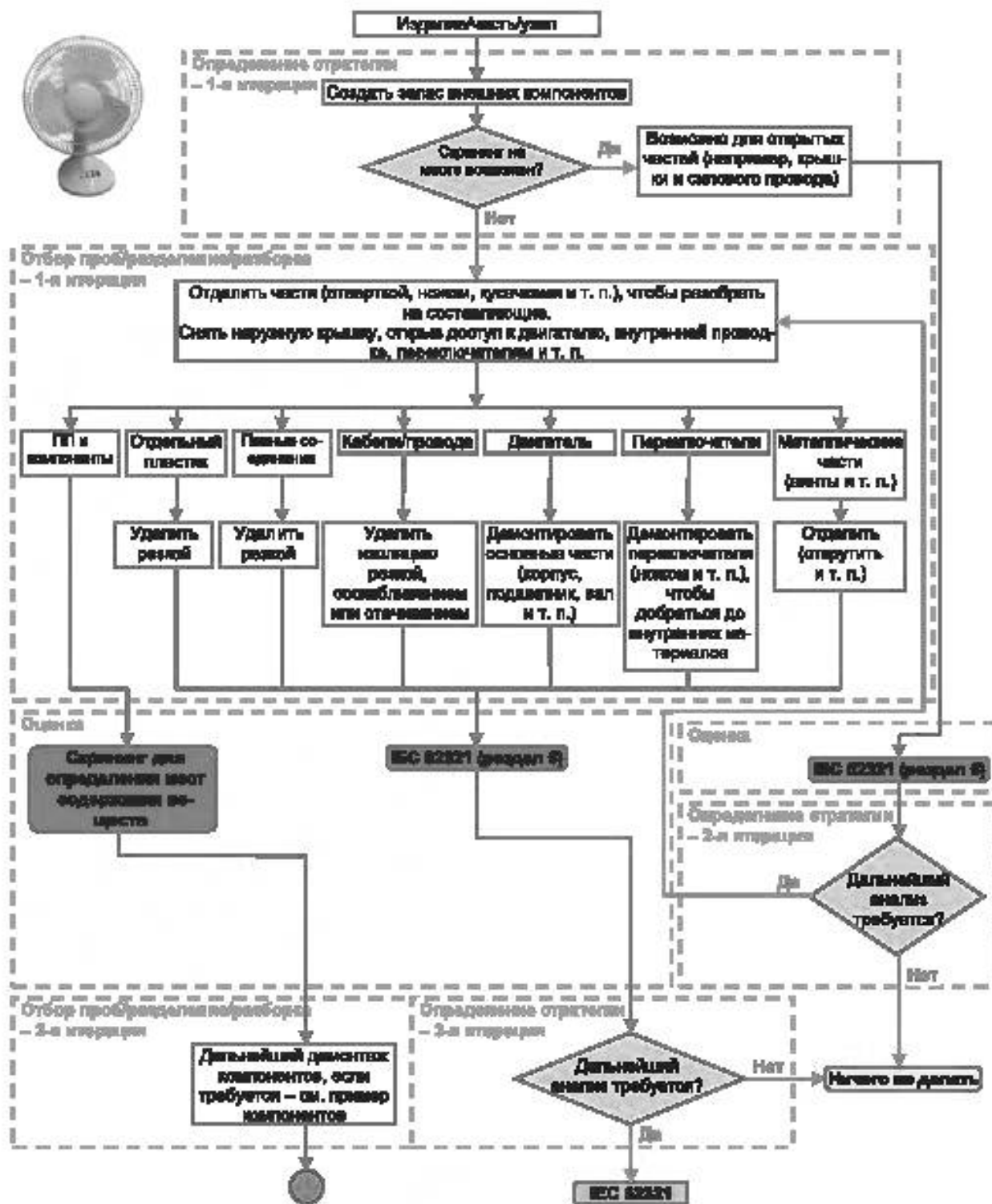
Рисунок А.6 — Отбор образцов настольного вентилятора
