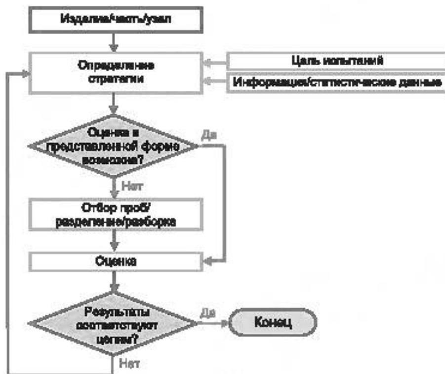
Рисунок 1 — Общая повторяющаяся процедура отбора образцов
