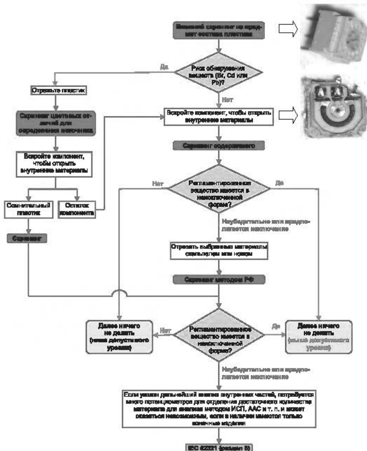
Рисунок А.8 — Отбор образцов компонентов — SMD потенциометр
