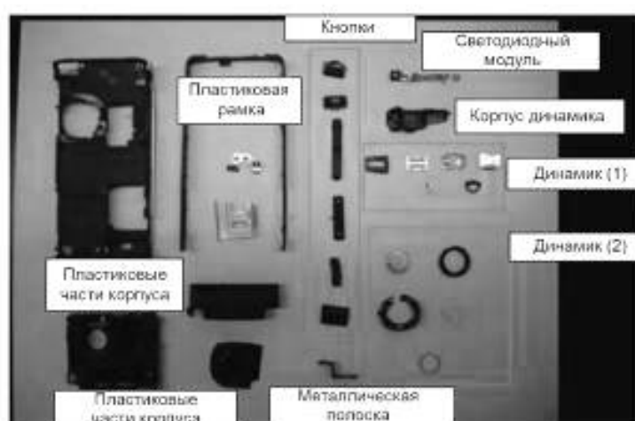
Рисунок Е.5 — Полная разборка нижней части корпуса
