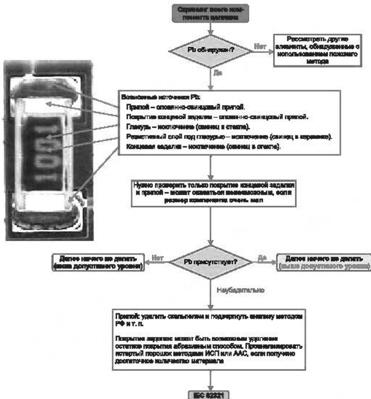
Рисунок А.7 — Отбор образцов компонентов — толсто пленочный резистор
