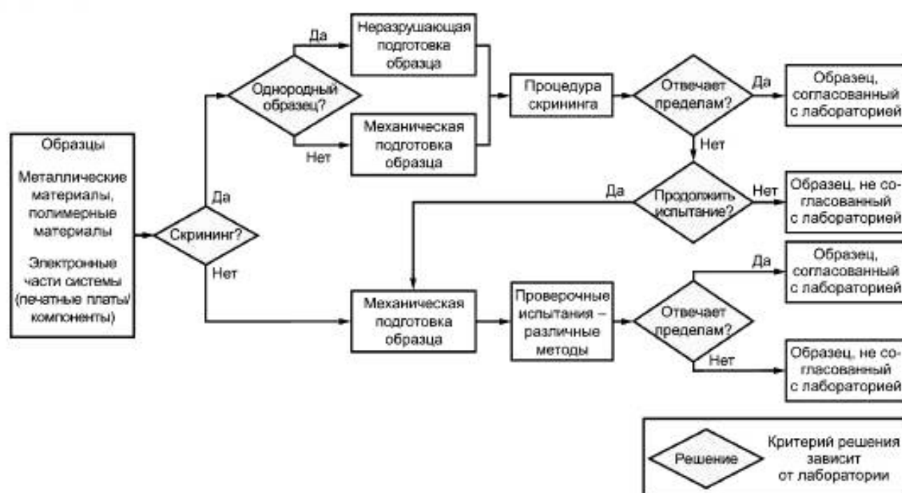
Рисунок 1 — Блок-схема проведения испытаний
