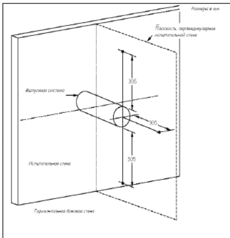
Рисунок 3 – Стена для проверки выпуска газов
