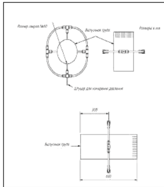
Рисунок 4 – Пьезо-кольцо и детали конструкции
