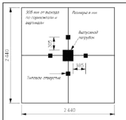
Рисунок 2 – Испытательная стена с указанием местоположений отверстий приема статического давления и выпускным патрубком
