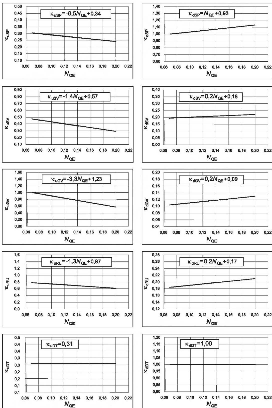
Рисунок В.8 — \kappa_{\text{исо}} и \kappa_{\text{дсо}} для каждого элемента насос-турбины при работе в турбинном режиме
