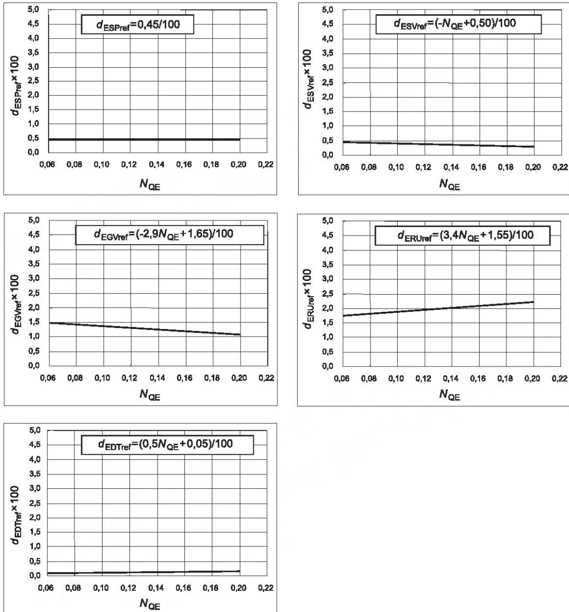
Рисунок В.12 — Нормализованные d_{ECOref} и d_{Eref} для насос-турбины в насосном режиме
