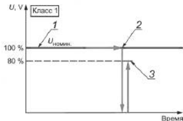
Рисунок A.3 — Разъяснения, касающиеся рабочего диапазона напряжений катушки
