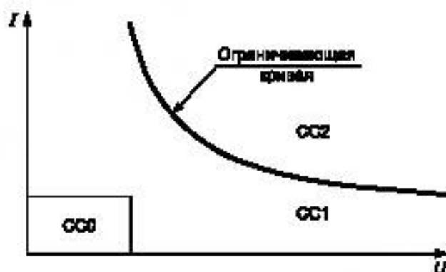
Рисунок С.3 — Категории контактных нагрузок
