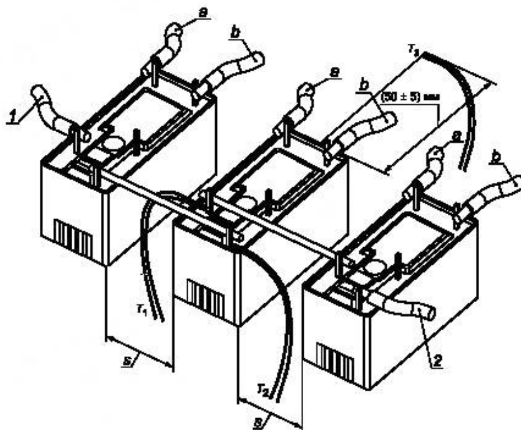
1, 2 — клеммы контактов; а, b — клеммы катушки; S — установочное расстояние; T_1 — термодатчики.
