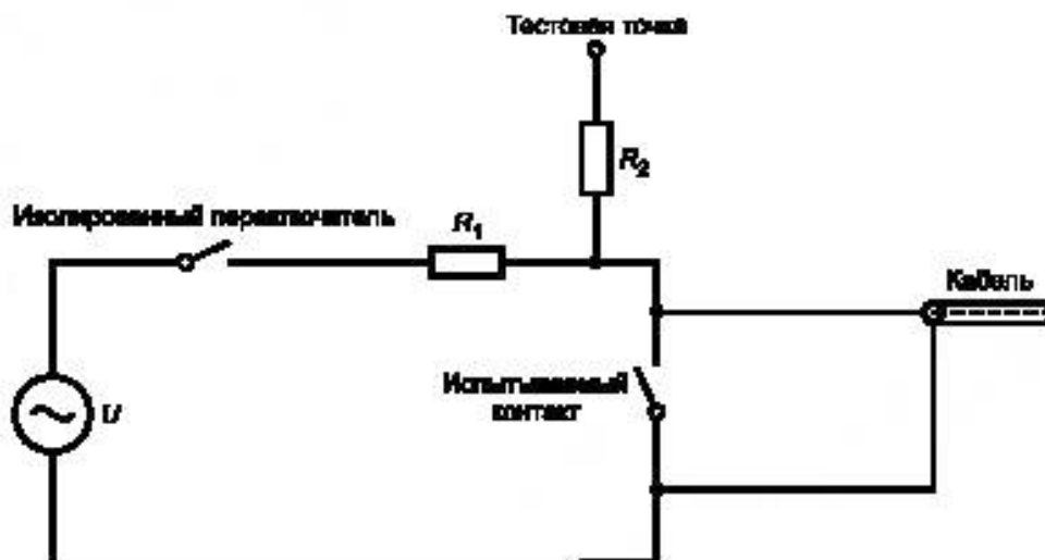
Рисунок D.1 — Схема для кабельной нагрузки
