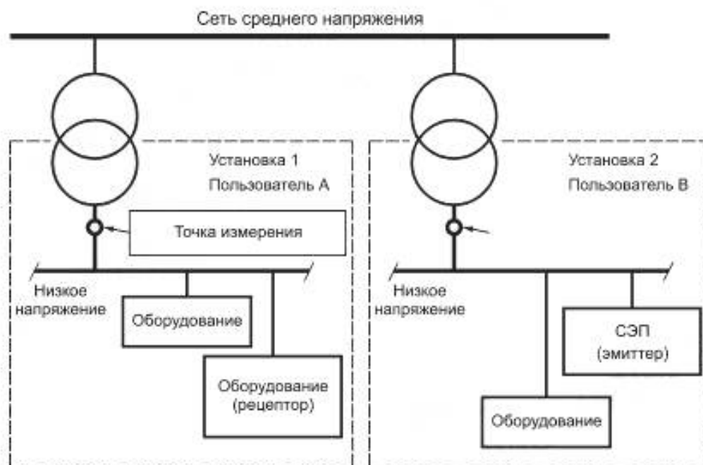
Рисунок 5 — Распространение помех
