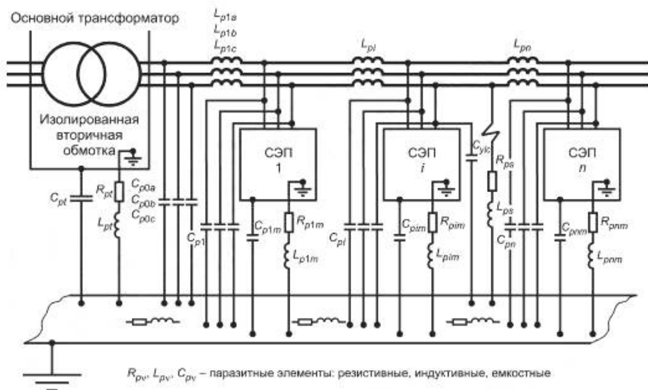
Рисунок D.3 — Безопасность и применение фильтров
