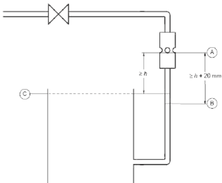
Рисунок 1 – Измерение расстояния h для трубопроводных прерывателей
