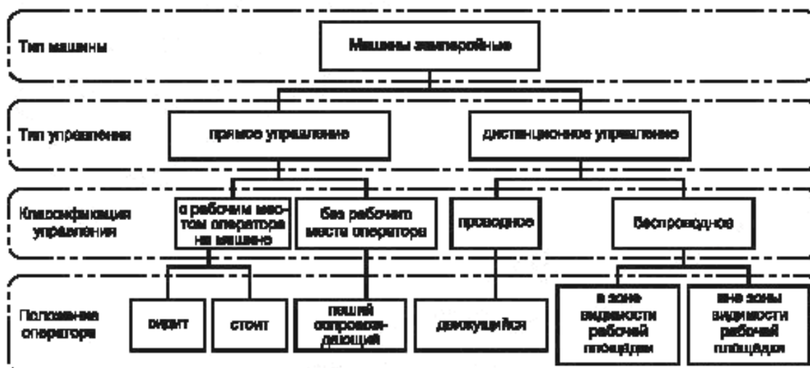
Рисунок В.1 — Варианты управления землеройной машиной
