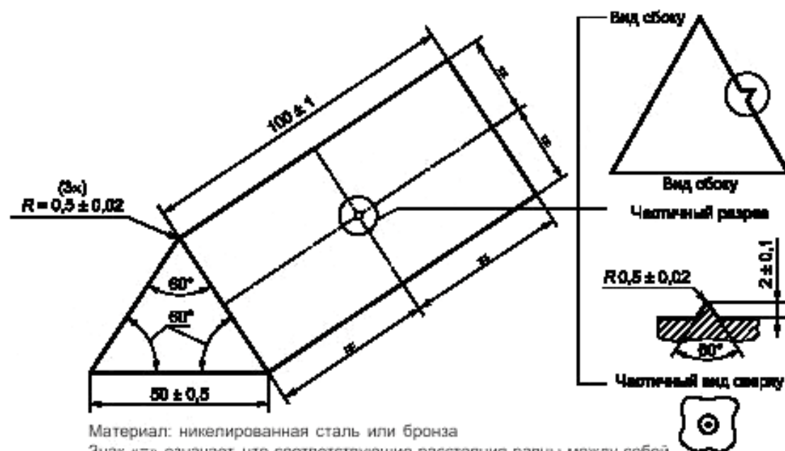
Рисунок 6а — Оправка
