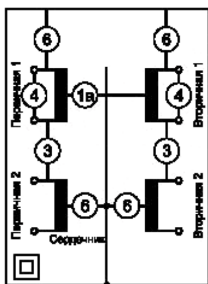
а) Сердечник, соединенный с корпусом
