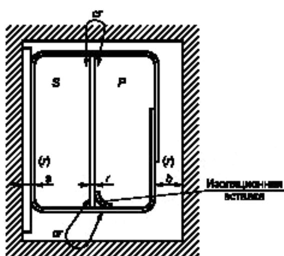
Первичная и вторичная обмотки, обернутые изоляционным материалом (нет путей утечки) Класс I (II) М.2.1 д)
