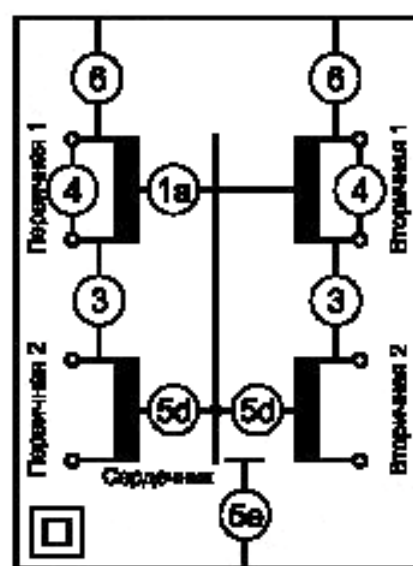
б) Сердечник, не соединенный с корпусом
