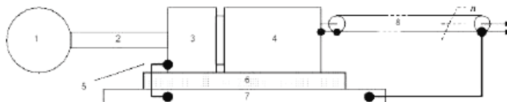
1 – рабочая среда; 2 – трубка; 3 – адаптер давления; 4 – датчик давления; 5 – заземление; 6 – изолирующая прокладка; 7 – эталонная земля; 8 – соединительные п. линии
