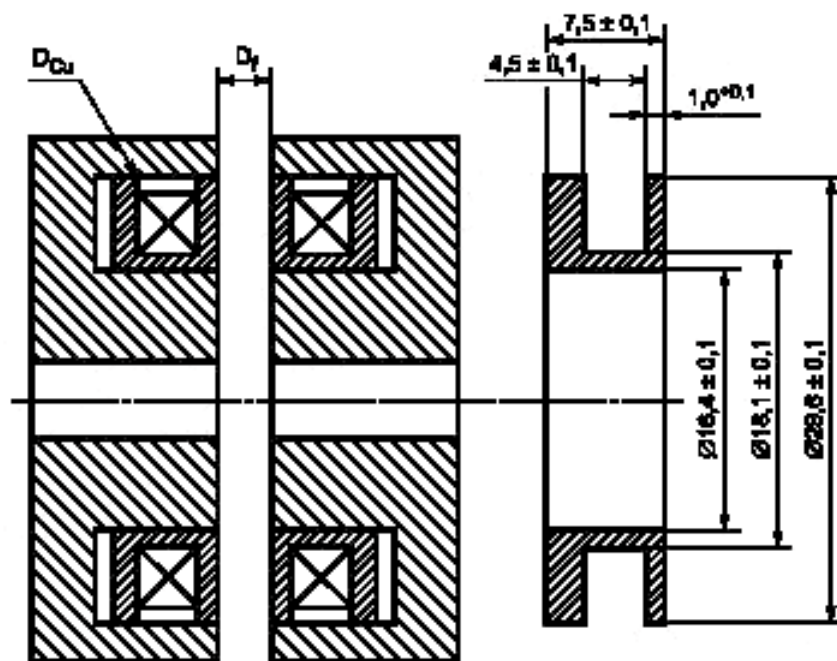
Ферритовый сердечник FP 26 x 22
