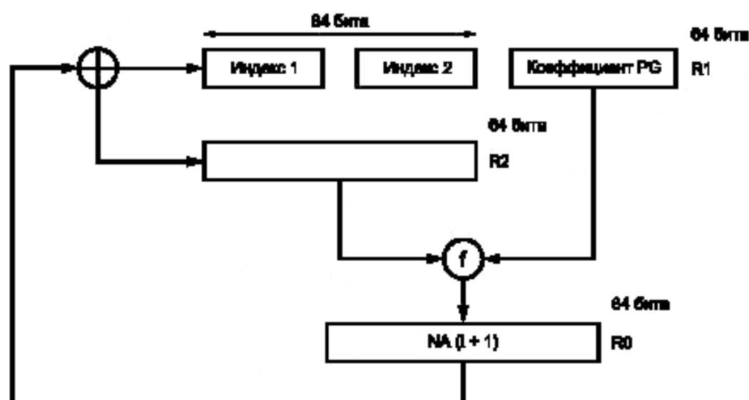
Блок-схема
