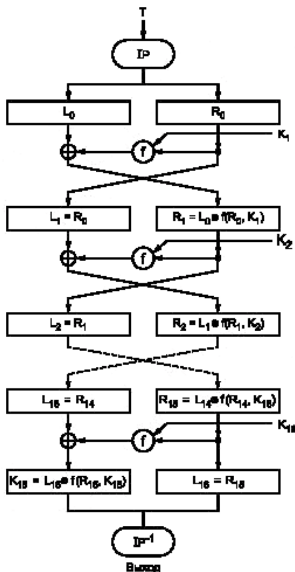
Блок-схема алгоритма кодирования DES
