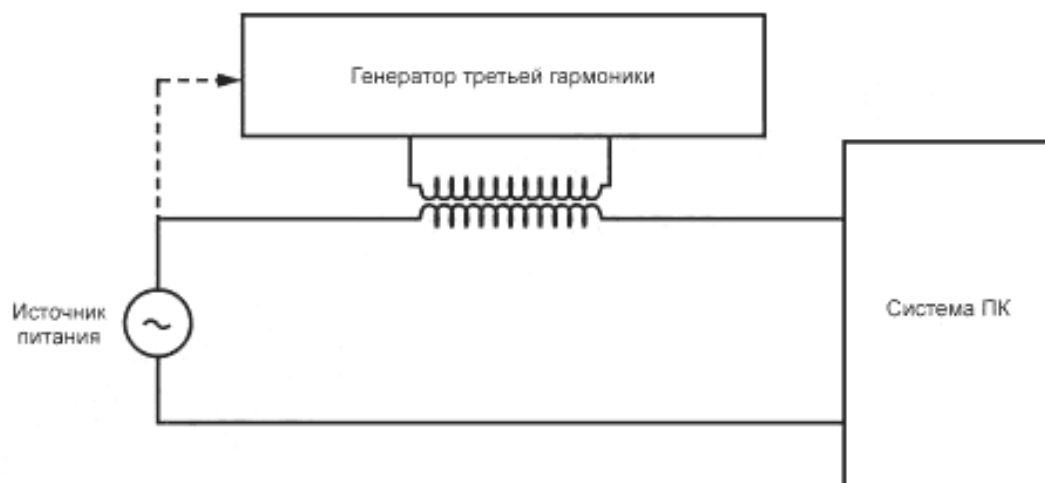
Рисунок 7 — Испытание на устойчивость к напряжению третьей гармоники
