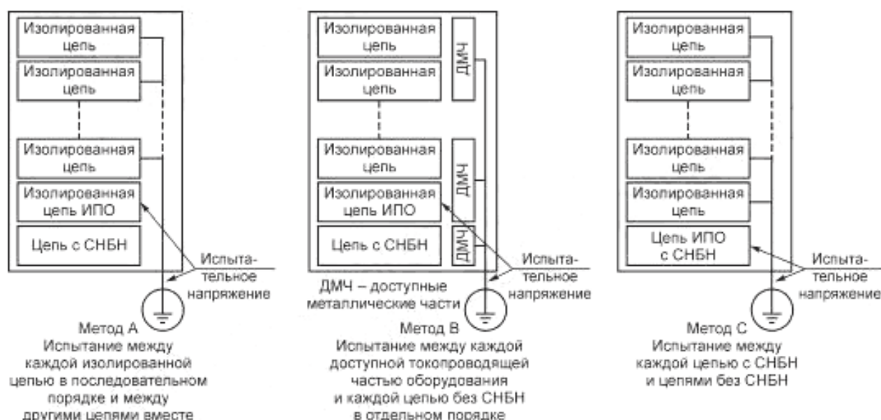
Рисунок 13 — Методы испытания на электрическую прочность диэлектрика
