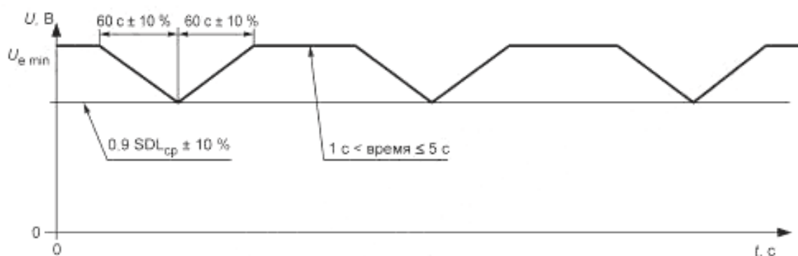
Рисунок 10 — Испытание на медленное изменение напряжения питания
