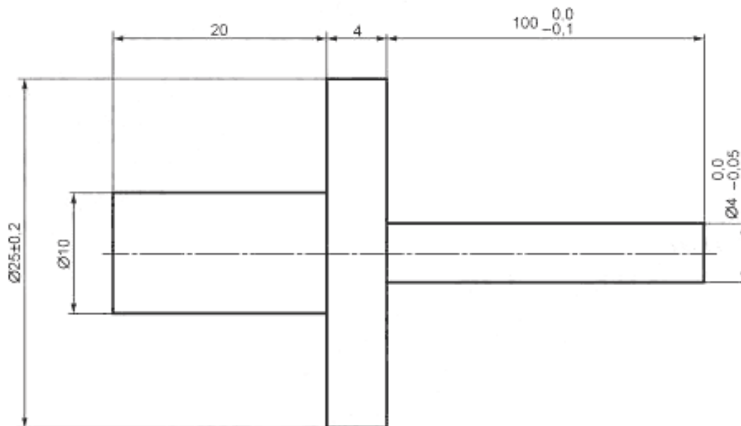
Рисунок С.3 — Испытательный штифт 100 × 4 мм
