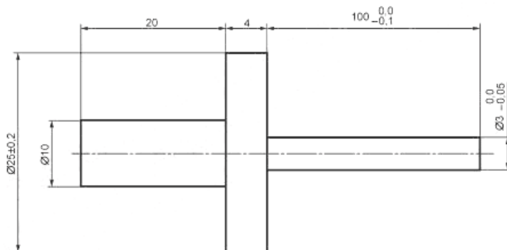
Рисунок С.4 — Испытательный штифт 100 × 3 мм
