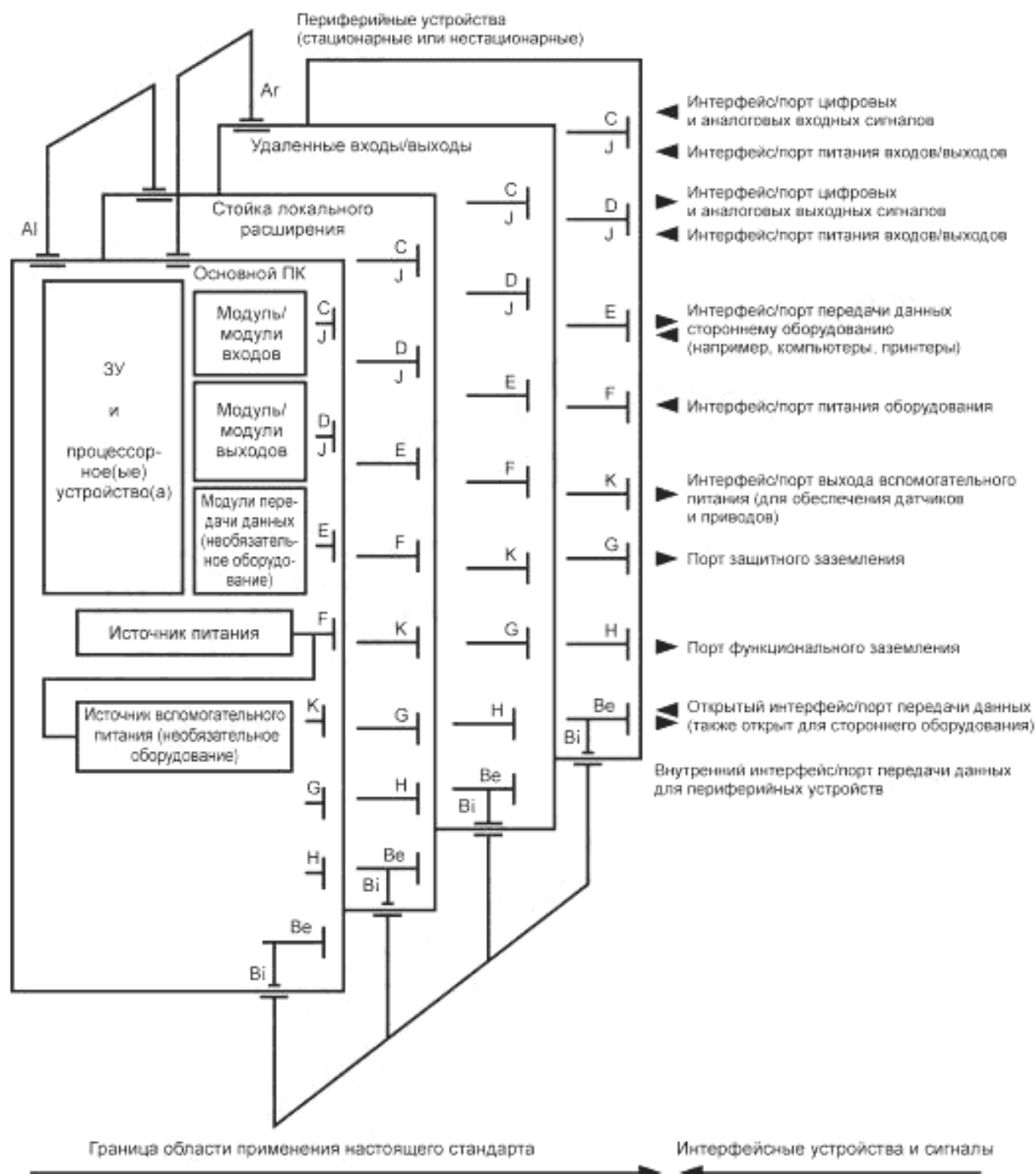
Рисунок 2 — Типовая конфигурация интерфейсов/портов системы ПК
