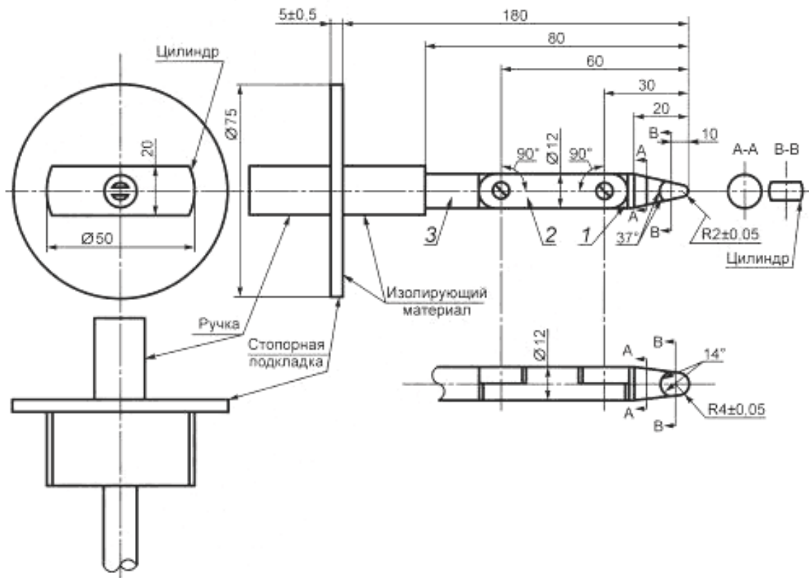
Рисунок С.1 — Шарнирный испытательный палец
