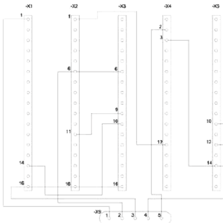
Рисунок 81 – Пример схемы соединений для субблока
