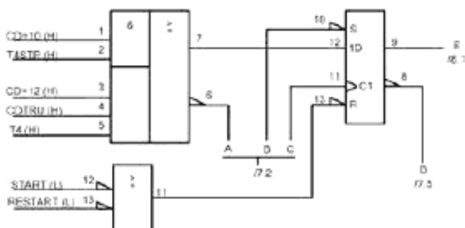
Рисунок 40 – Деталь принципиальной схемы, в которой используется указатель полярности логики
