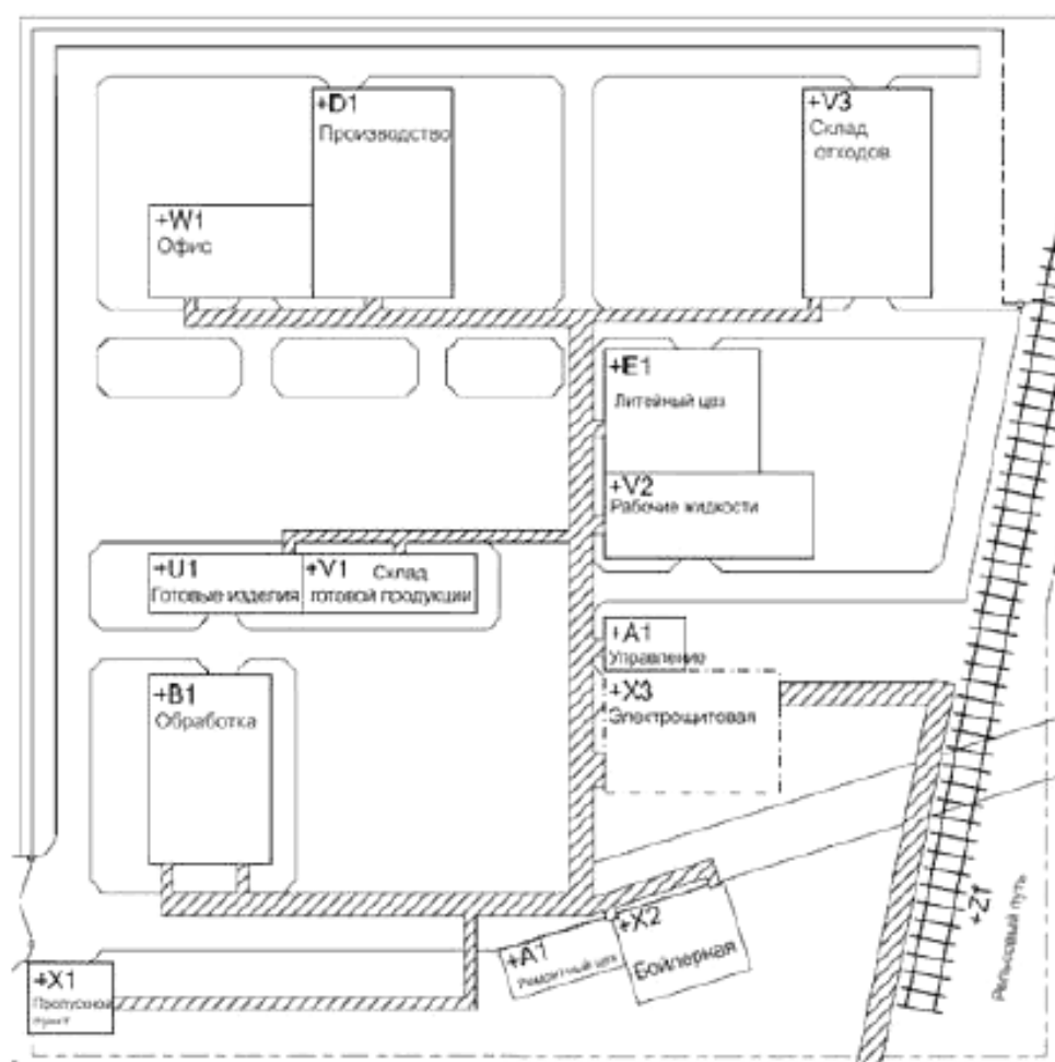
Рисунок 87 – Компоновочный чертеж промышленного предприятия
