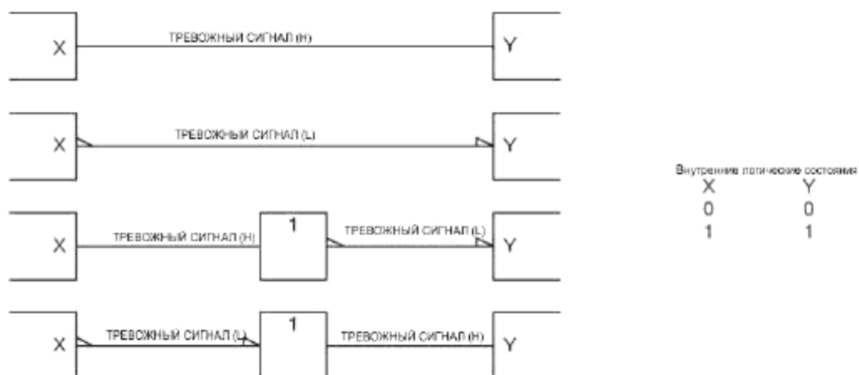
Рисунок 75 - Примеры использования указателя полярности логики
