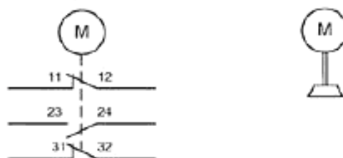
Рисунок 32 – Пример представления механических связей
