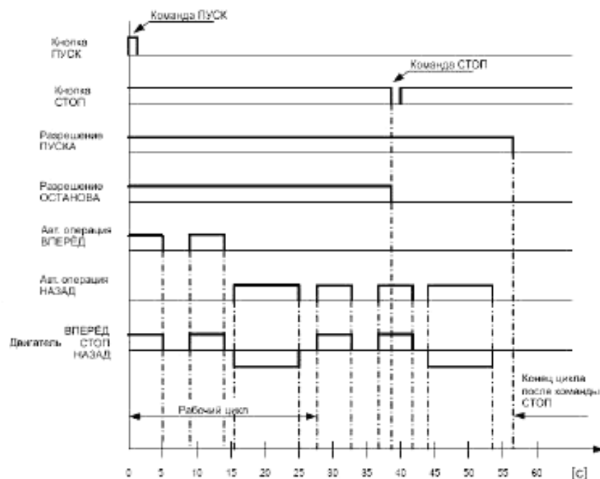
Рисунок 93 – Пример временной диаграммы
