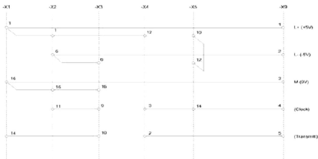
Рисунок 82 – Пример упрощенного представления схемы соединений
