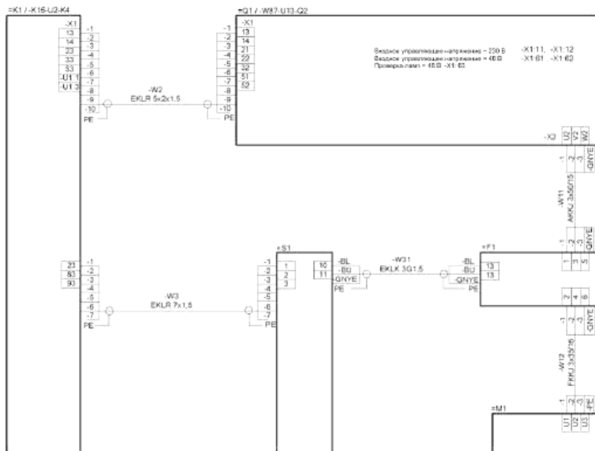
Рисунок 78 – Пример схемы соединений
