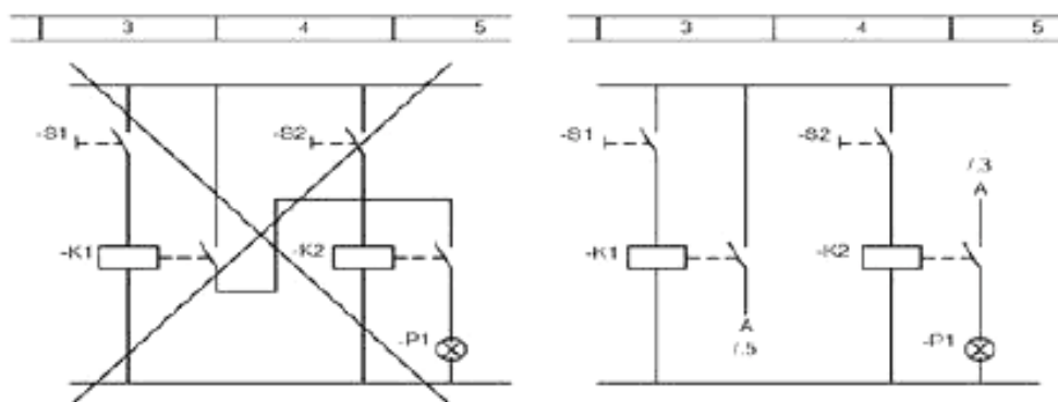
Рисунок 33 – Пример предотвращения изгибов и перекрещиваний
