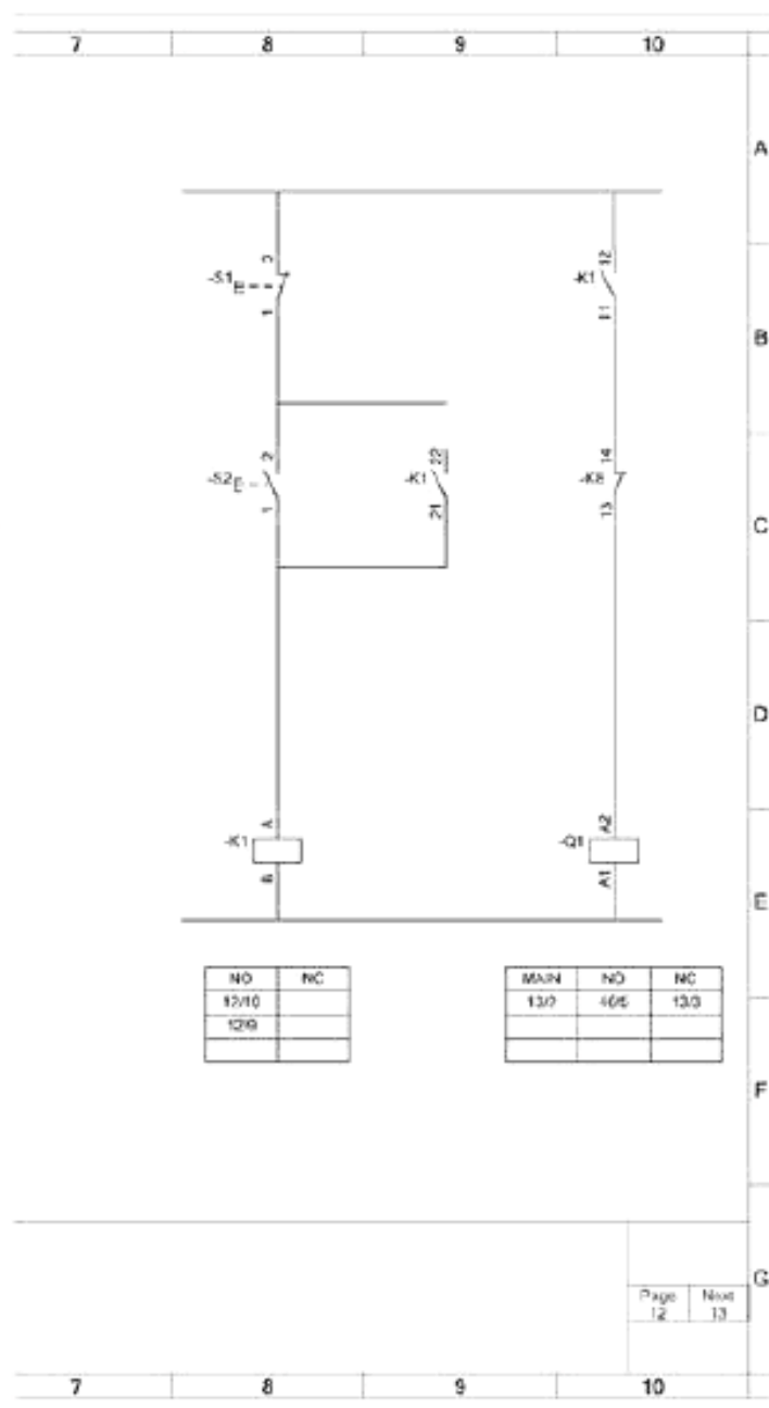
Рисунок 65 – Пример использования вставных таблиц
