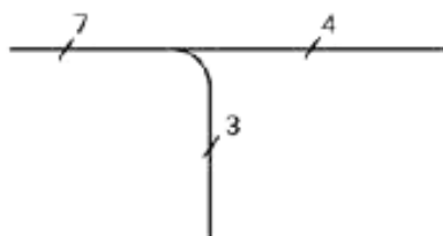
Рисунок 31 – Пример сочленения соединительных линий, представляющих жгуты проводов
