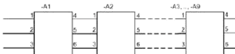
Рисунок 24 – Упрощенное представление последовательного соединения идентичных объектов
