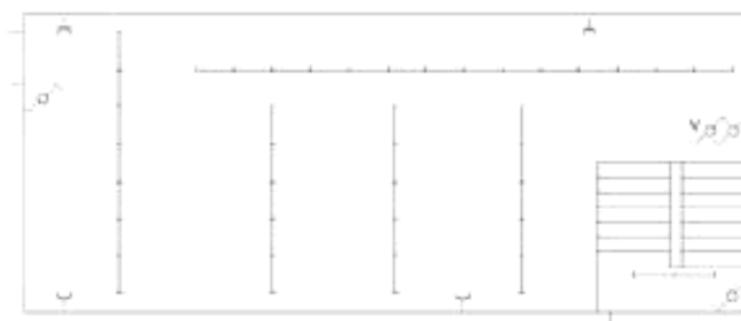
с) Базовый чертёж с добавлением устанавливаемых светильников
