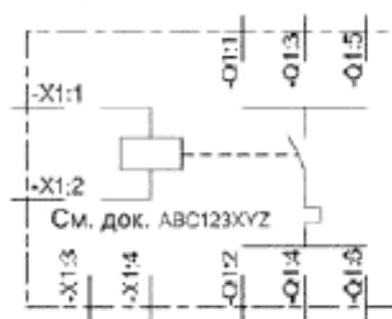
Рисунок 94 – Пример схемного представления пускателя двигателя
