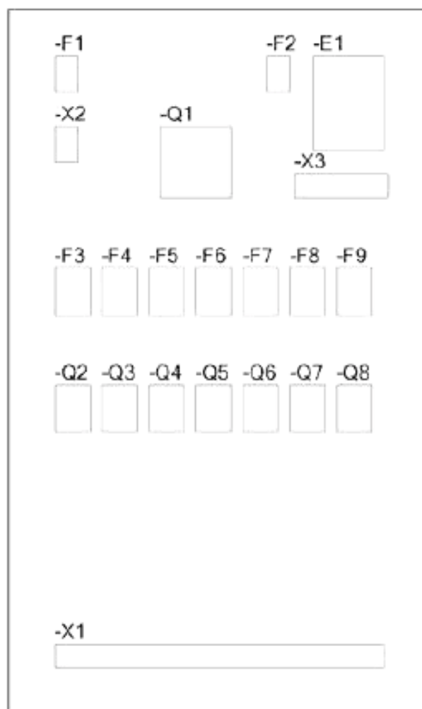
Рисунок 86 – Компонировочный чертеж монтажной панели шкафа
