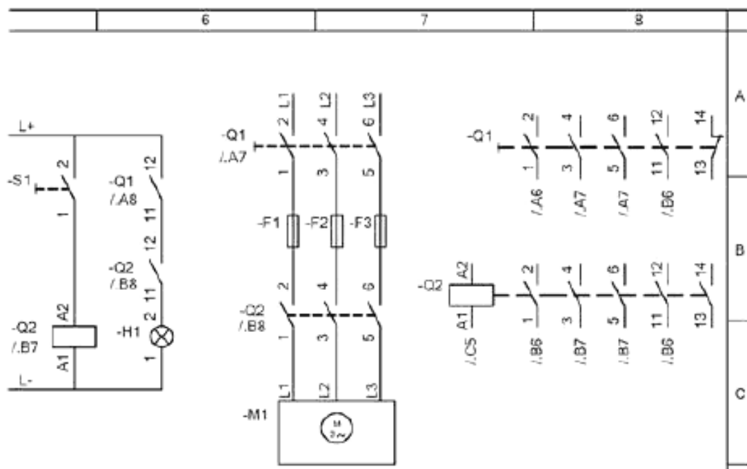
Рисунок 64 – Разъединенное отображение символических обозначений
