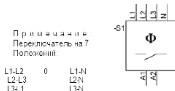
Рисунок 16 – Пример пояснительного примечания
