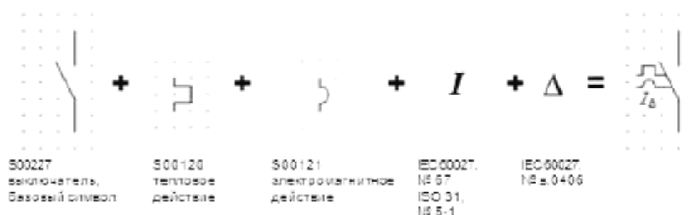
Рисунок А.9 – Символическое представление автоматического микровыключателя с устройством остаточного тока, вариант 3
