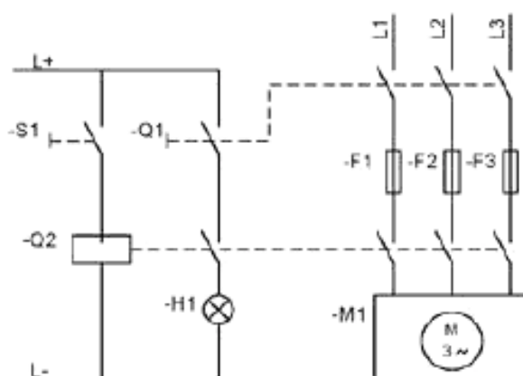
Рисунок 63 – Соединенное отображение символов
