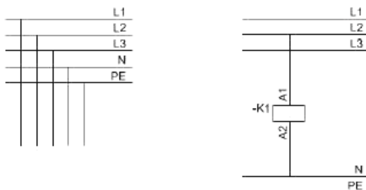
Рисунок 73 – Представление питающих цепей переменного тока
