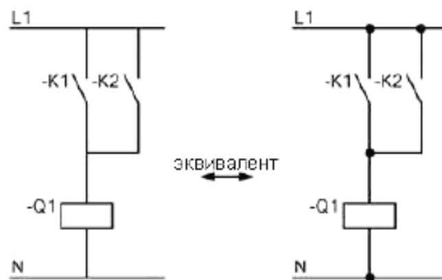
Рисунок 29 – Примеры сочленения соединительных линий
