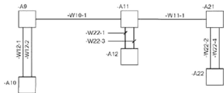
Рисунок 43 - Примеры ссылочных обозначений, ассоциируемых с соединительными линиями
