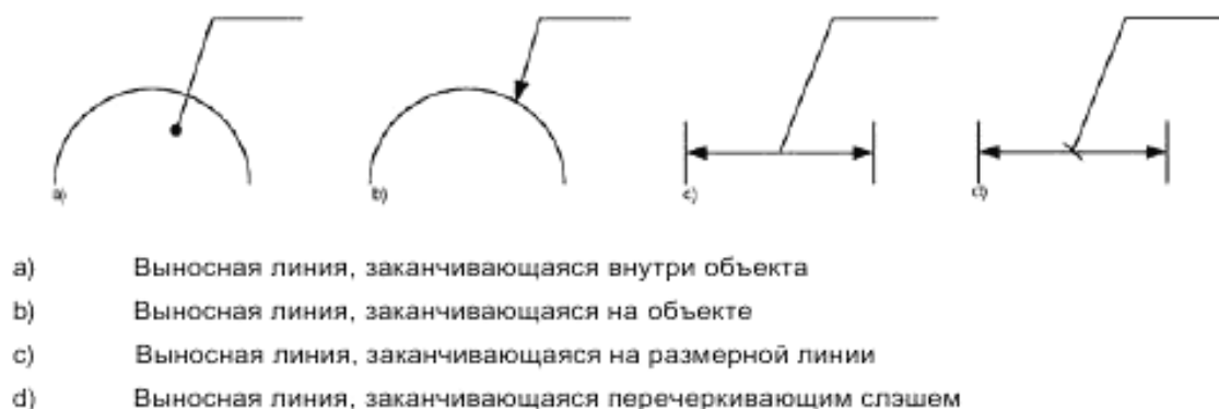
Рисунок 14 – Примеры выносных линий (из ISO 128-22)
