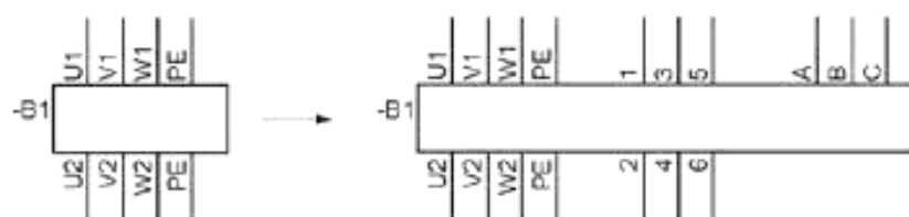
Рисунок 11 – Пример расширения символического обозначения
