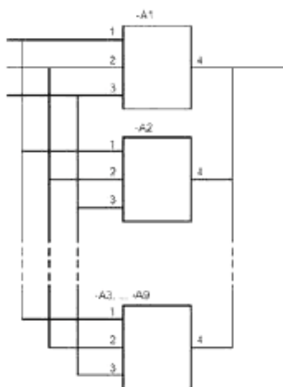
Рисунок 23 – Упрощенное представление параллельного соединения идентичных объектов
