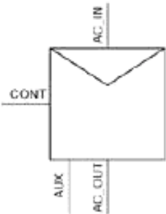
Рисунок 97 – Символ пускателя электродвигателя, предназначенный для использования в однолинейных представлениях
