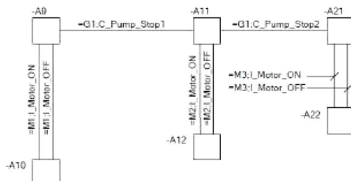
Рисунок 50 – Примеры обозначений сигналов, ассоциированных с соединительными линиями
