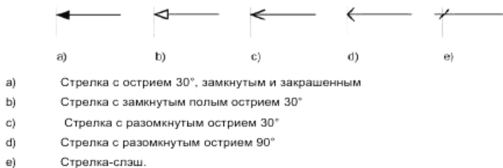
Рисунок 13 – Концевые элементы размерных линий (из ISO 129)
