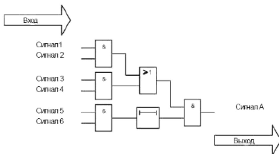
Рисунок 58 – Поток сигналов на функциональной схеме
