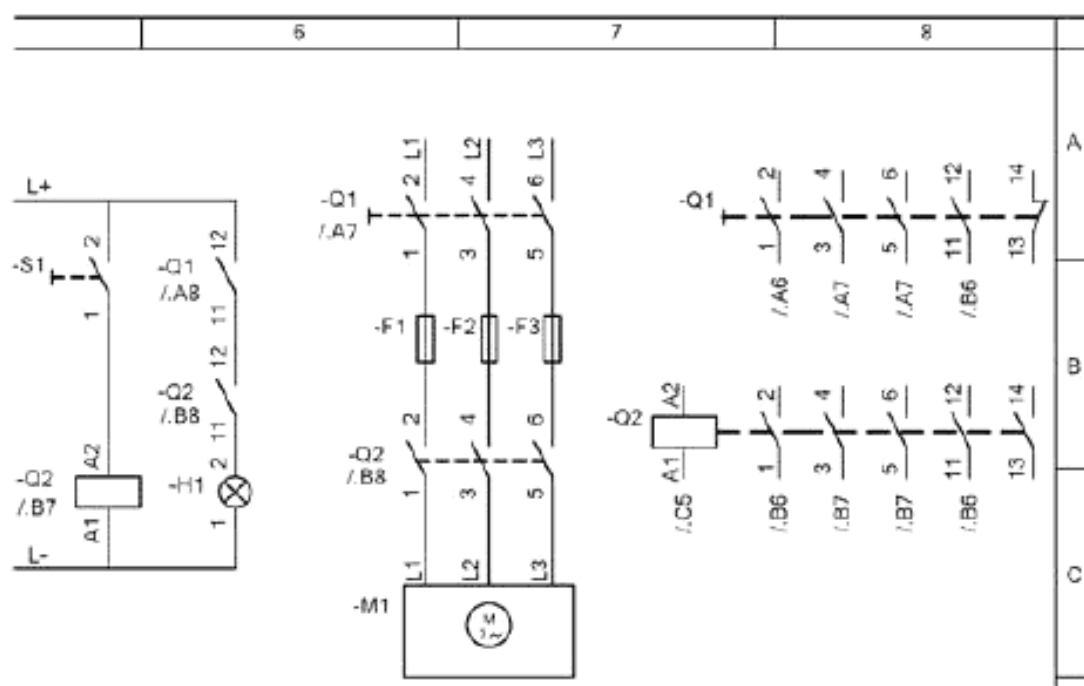
Рисунок 64 – Разъединенное отображение символических обозначений
