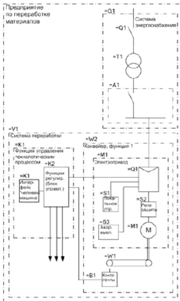
Рисунок 55 – Общая схема одной функции ленточного конвейера (пример взят из IEC 61346-1)
