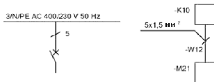
Рисунок 35 – Примеры связывания технических данных с соединительными линиями
