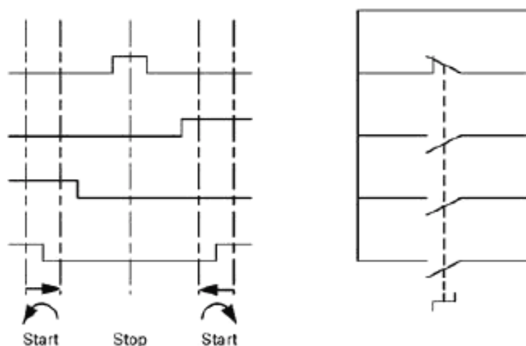
Рисунок 69 – Символическое обозначение переключателя, дополненное графическим представлением
