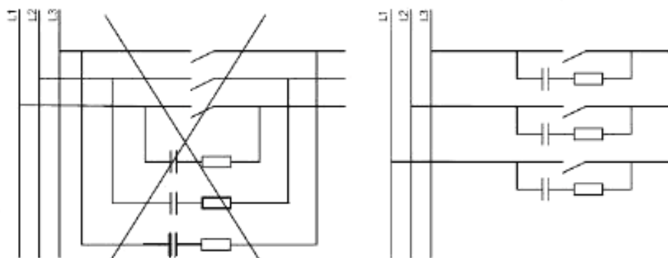
Рисунок 62 – Группирование символов функционально связанных компонентов
