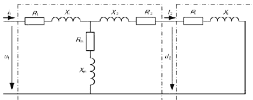
Рисунок 59 – Пример эквивалентной схемы электрической цепи
