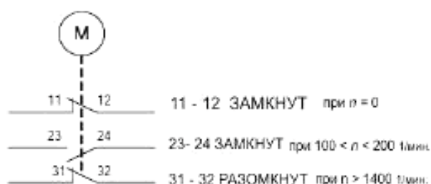
Рисунок 71 – Символ автоматического выключателя, снабженный пояснением
