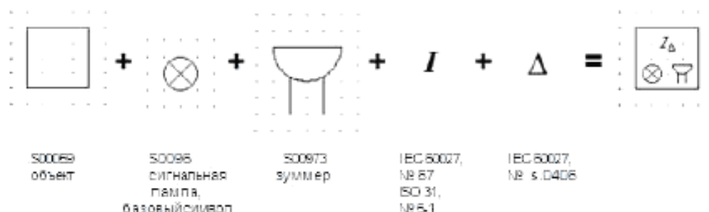
Рисунок A.11 – Пример символа для представления RCM
