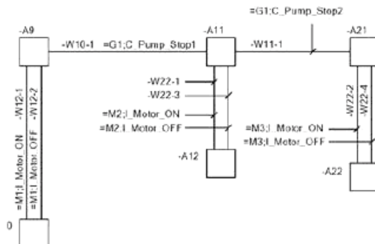
Рисунок 51 – Примеры ссылок обозначений и обозначений сигналов, ассоциируемых с соединительными линиями
