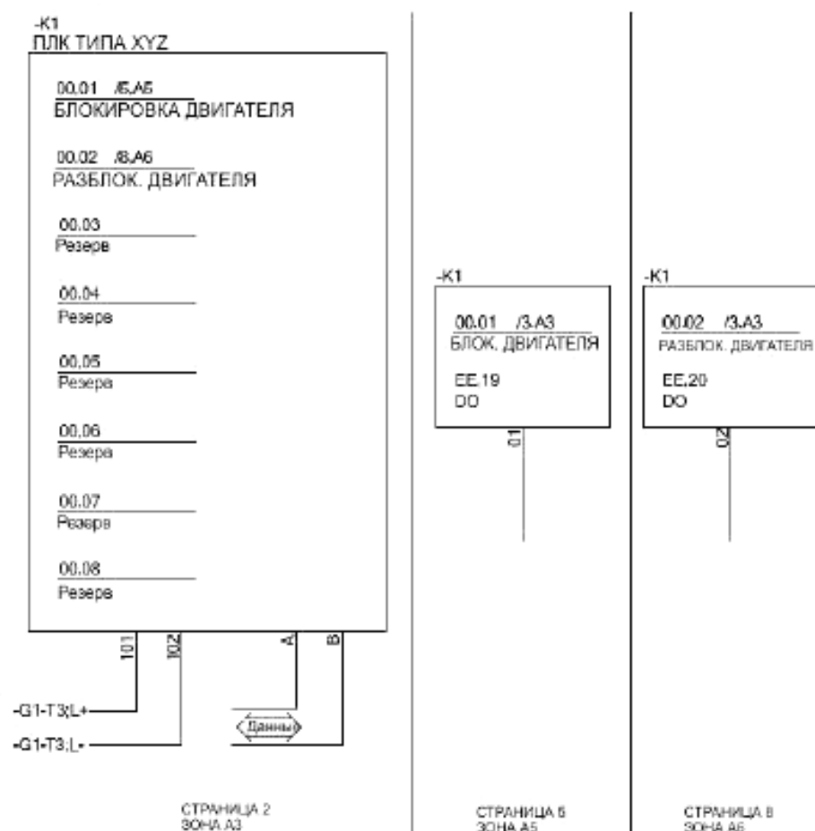
Рисунок A.12 – Символические представления для ПЛК
