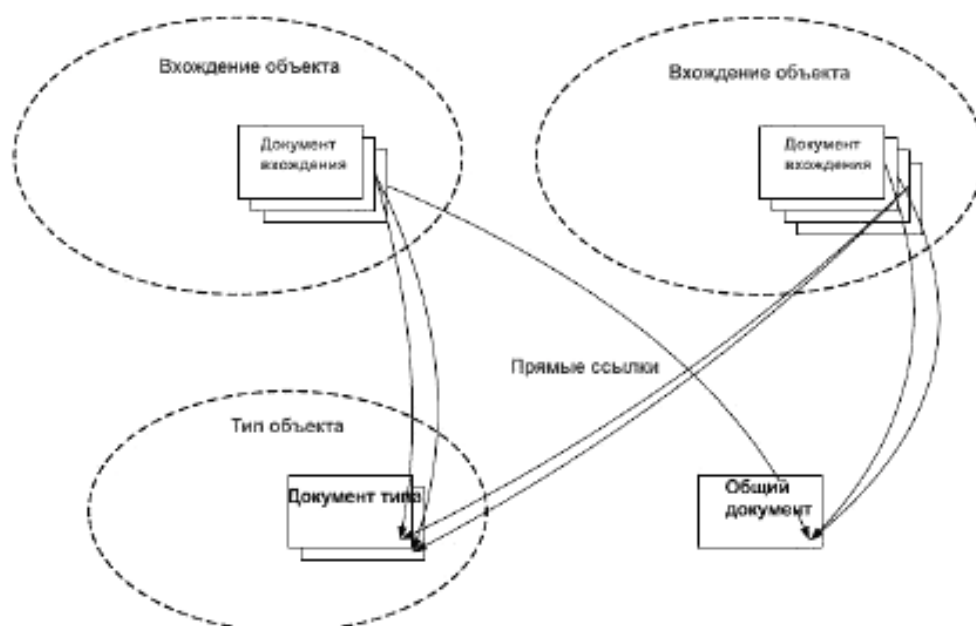
Рисунок 100 – Прямые ссылки
