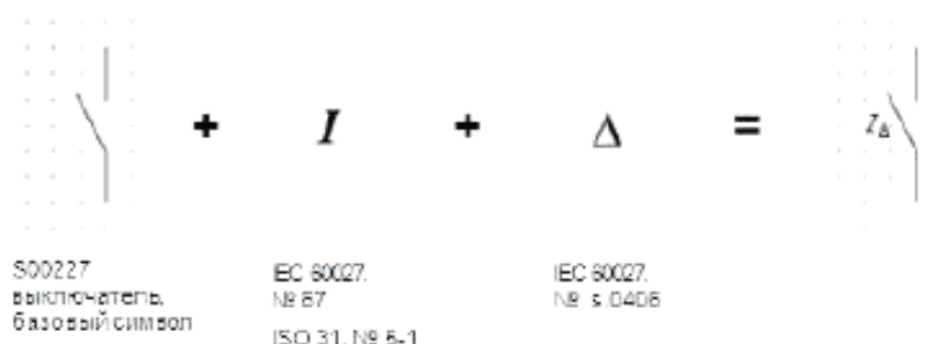
Рисунок A.10 – Пример символа для представления RCD
