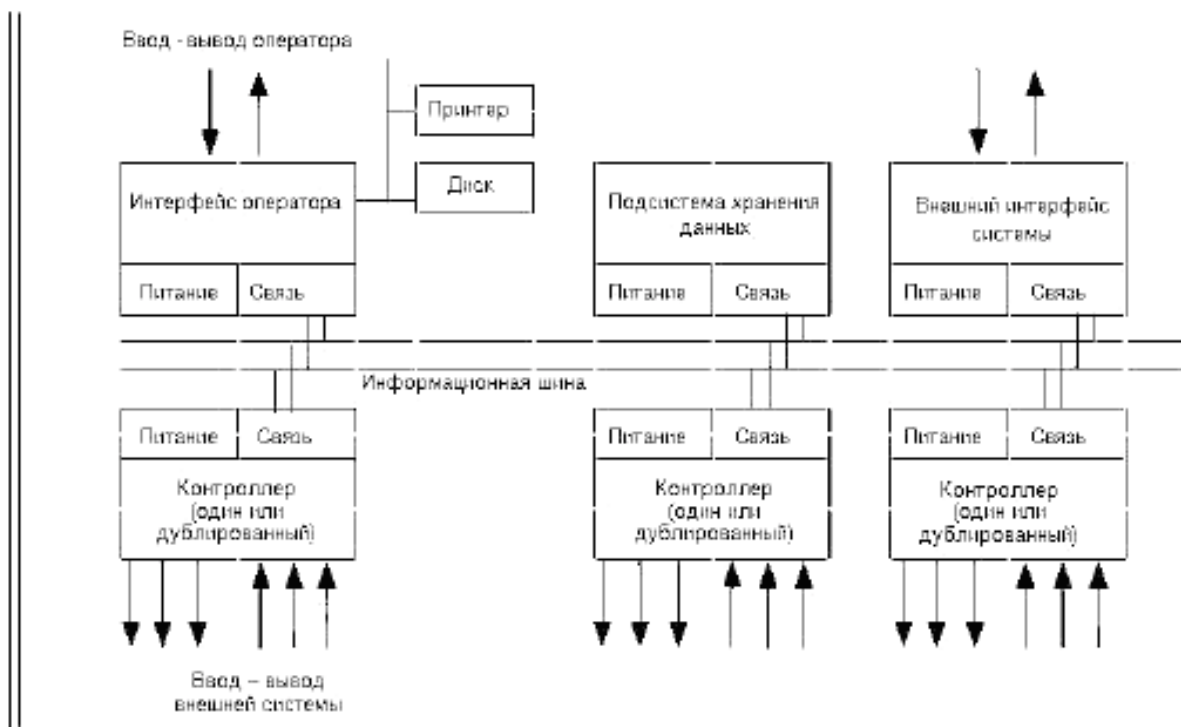
Рисунок С.2 — Общая физическая модель системы
