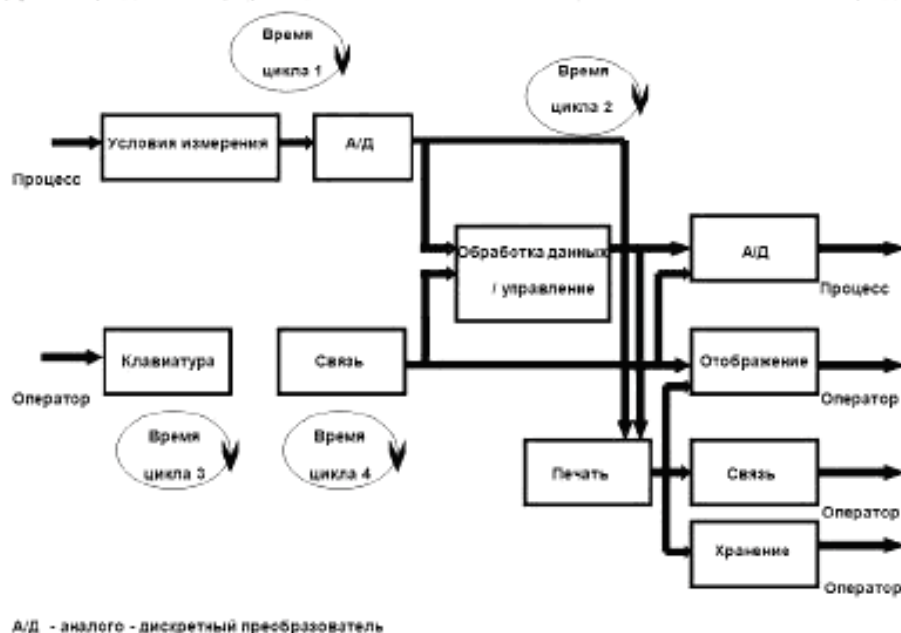
Рисунок С.1 — Схематическая функциональная диаграмма системы
