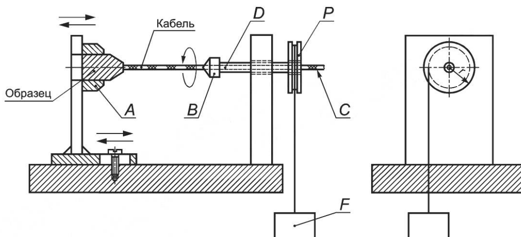
А — устройство крепления образца; В — устройство крепления провода; С — конец провода; D — вращающийся вал (полюс); r — радиус шкива; F — груз; крутящий момент F \cdot r ; P — шкив
