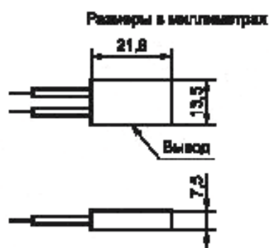
Рисунок 5 — Размеры свинцового вывода
