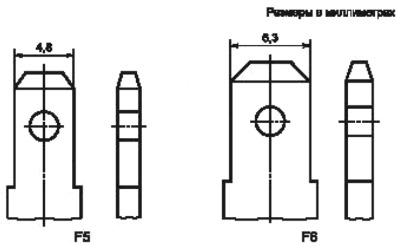
Рисунок 3 — F-контакты (плоские контакты)
