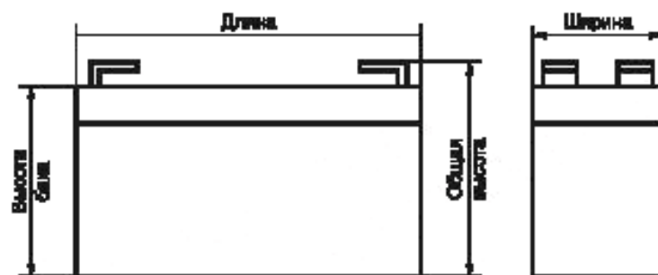
Рисунок 1 — Батареи призматического типа (Р-тип)
