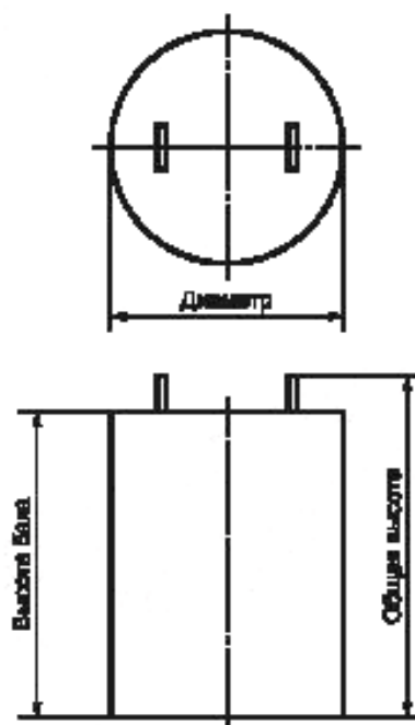
Рисунок 2 — Аккумуляторы цилиндрического типа (С-тип)
