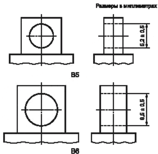
Рисунок 4 — В-контакты (болтовое соединение)
